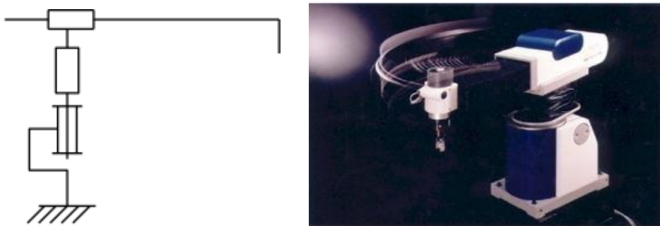
Figure I.9 : Robot cylindrique(Seiko) [28].
