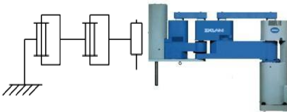
Figure I.8 : Robot SCARA (Sankyo) [28]
