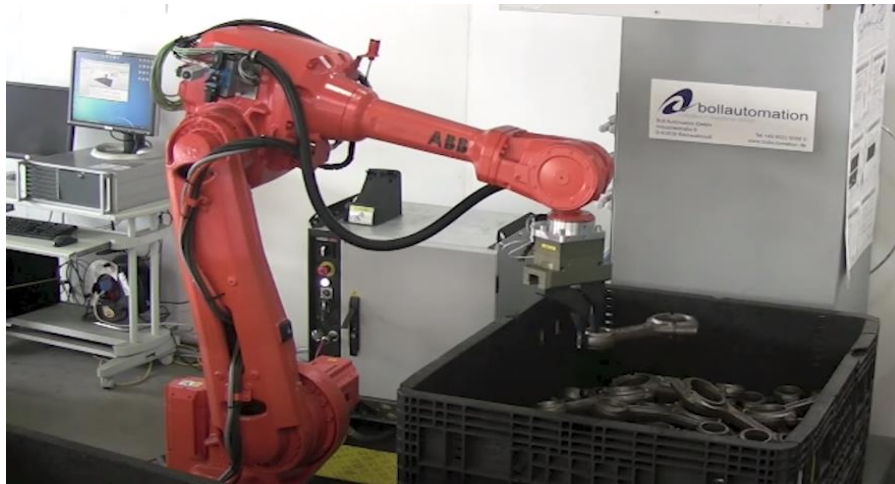
Figure II.4: Robot industriel de la manipulation des pièces [29].
