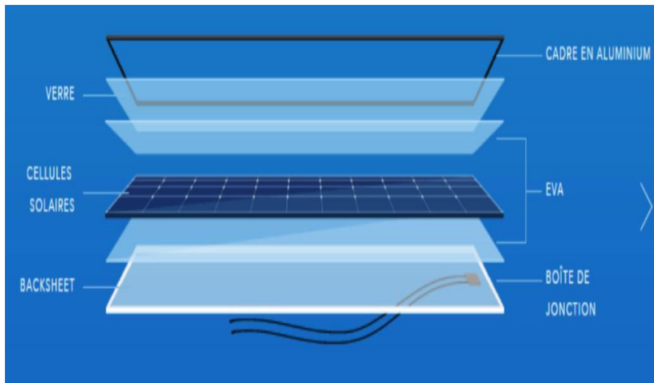
Fig. I.9 Constitution d'une cellule photovoltaïque
