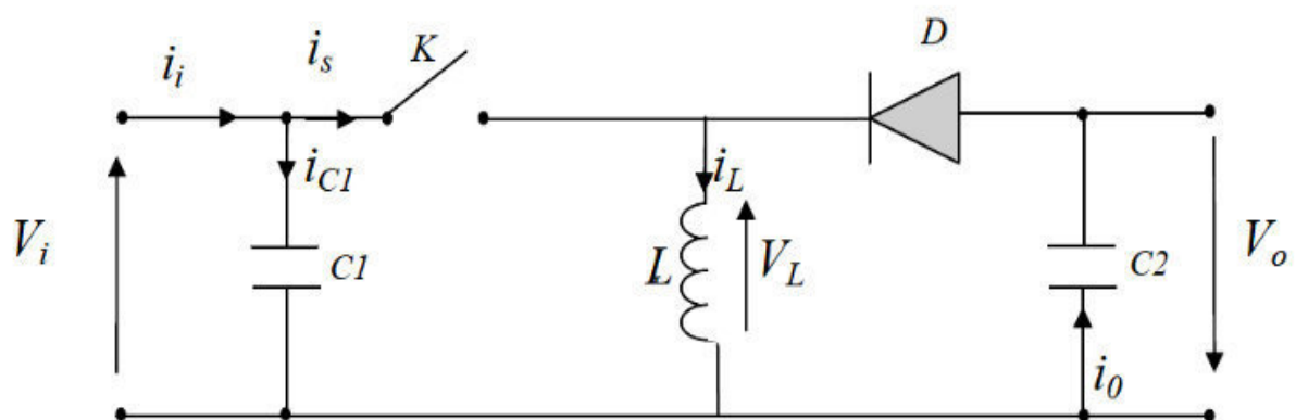
Fig. III.2 Schéma de principe d'une alimentation à découpage.
