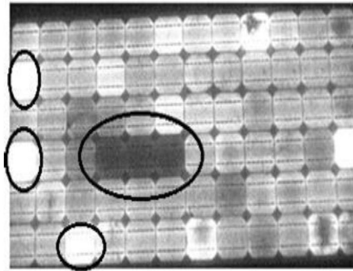
Fig.II.16 Image de la surface d'un module PV obtenue par électroluminescence
