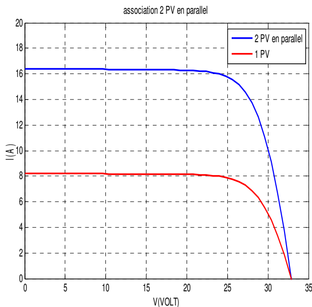
Fig. I.20 : Caractéristique I(V) pour une association de cellules en parallèle
