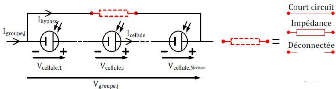
Fig. II.11 Schéma d'un groupe de cellules PV en série avec la diode by-pass défailante.
