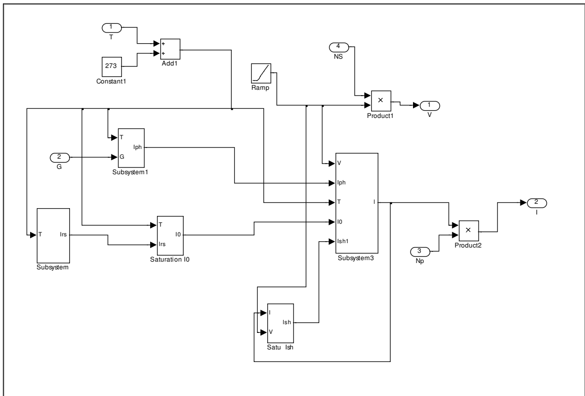
Fig.(II.7) schéma Schéma Simulink de simulation du champ PV
