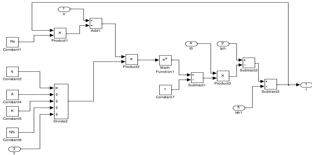
Figure (II.6 )Schéma Simulink pour simulation du courant I
