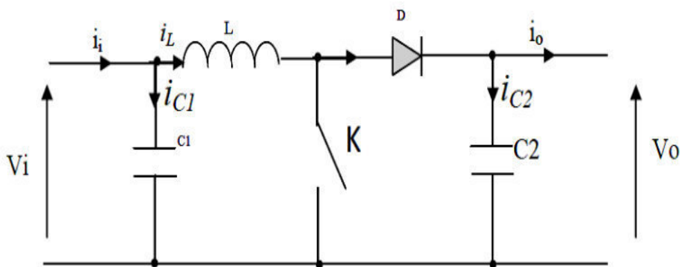
Fig. III.7 : Schéma de principe d'un convertisseur Boost.
