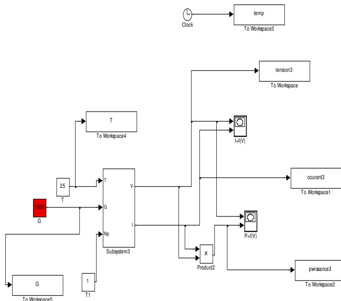
Fig. IV.13 Schéma de simulation pour obtenir les caractéristiques (I-V) et (P-V) d'un module photovoltaïque pour différentes températures.
