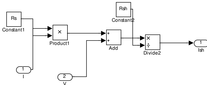
Fig.( II.4) Schéma Simulink pour simulation du courant I_{sh}
