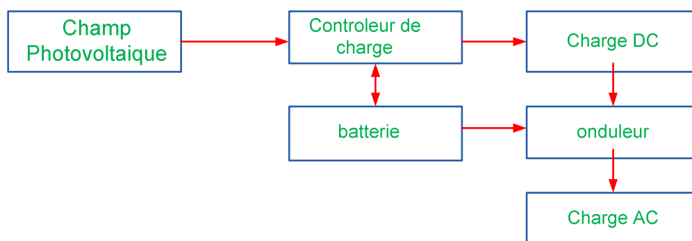
Fig. I.16 : Schéma d'installations autonomes.
