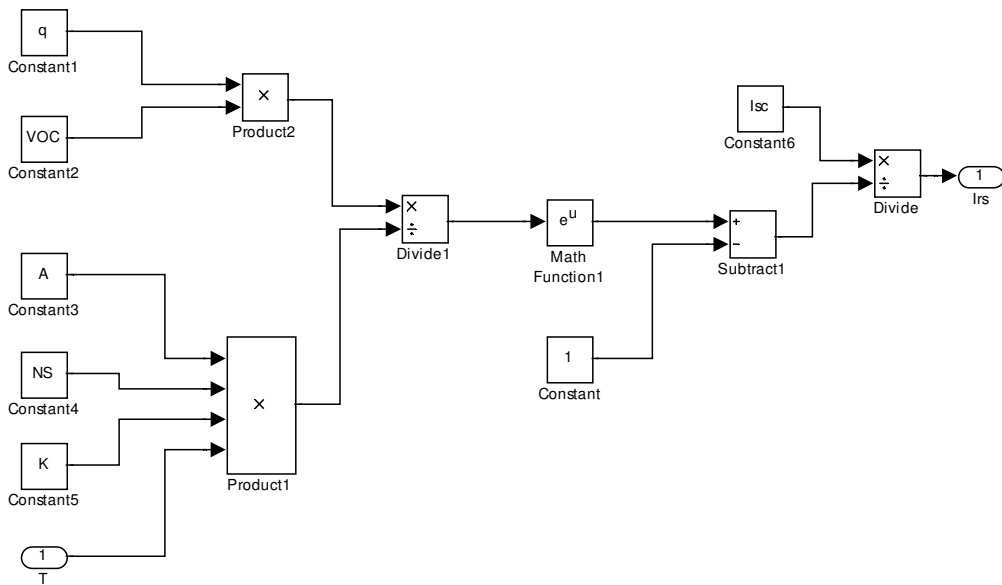
Fig. (II.3) Schéma Simulink pour simulation du courant I_{rs}
