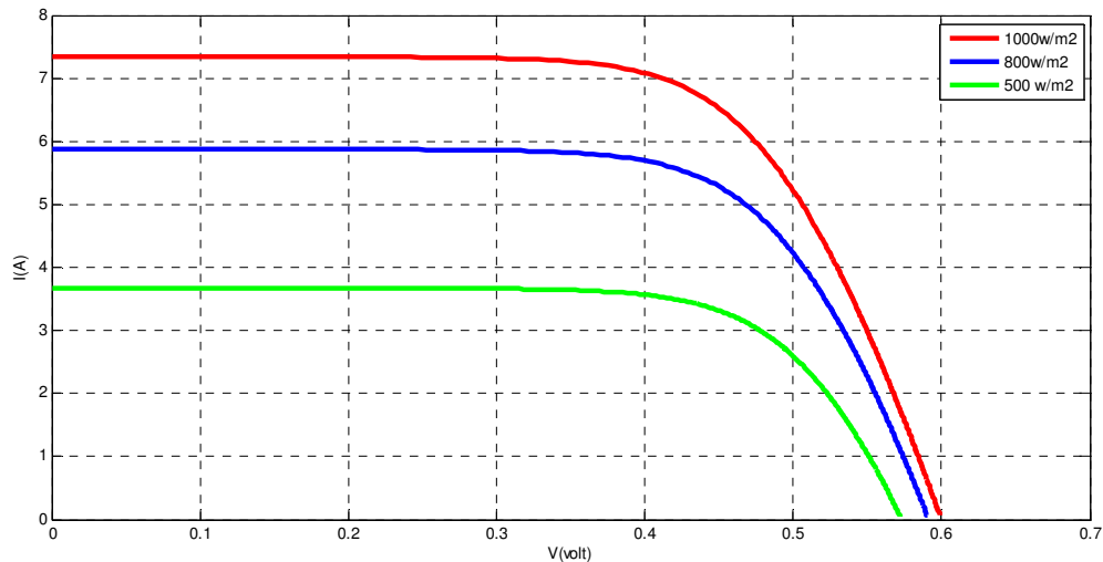
Fig. IV-2 Courbes I-V pour différentes valeurs de l'éclairement de la cellule.
