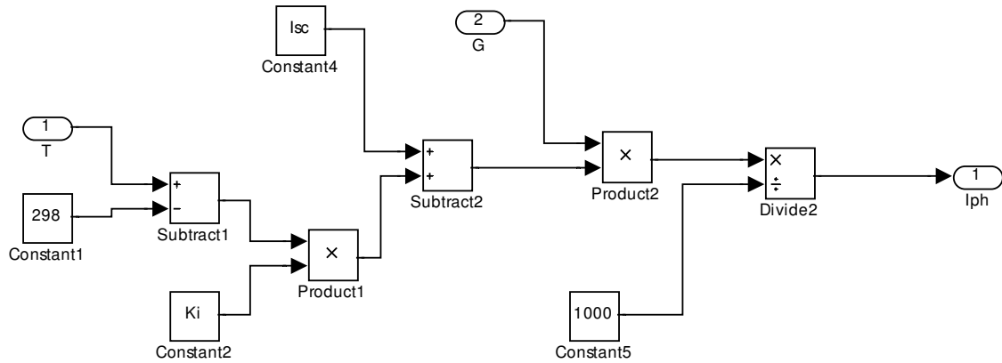
Fig.( II.2) Schéma Simulink pour simulation du courant I_{ph} .
