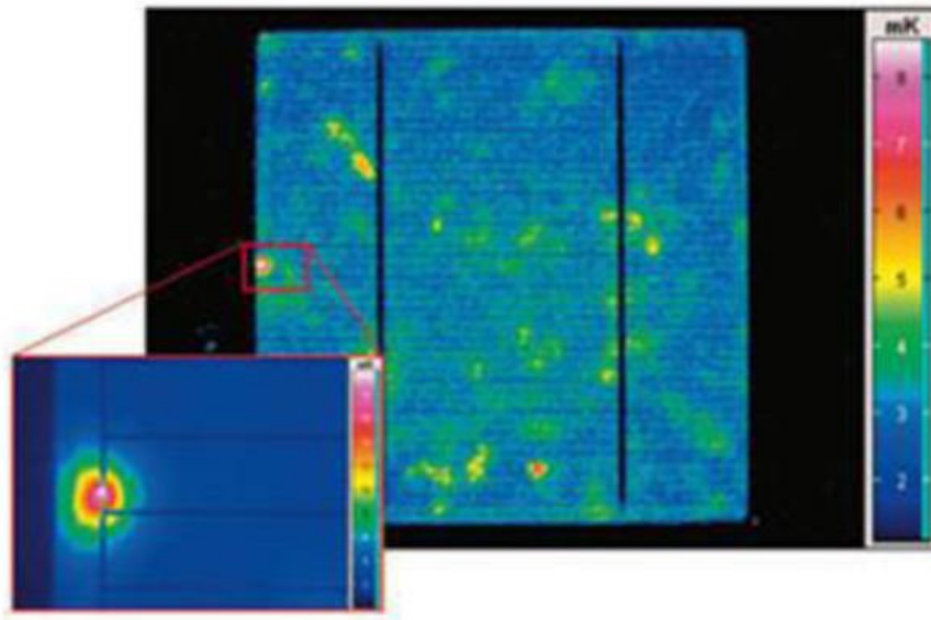
Figure II.15 Image thermographique d'une cellule PV en silicium.
