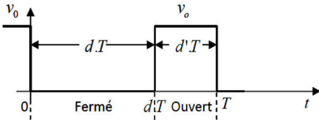
Fig. III.4 Durées de fermeture et d'ouverture d'un commutateur
