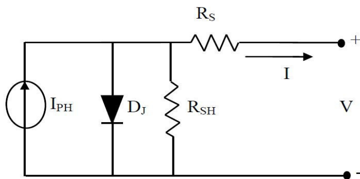
Fig.(II.1). Modèle à 1 diode
