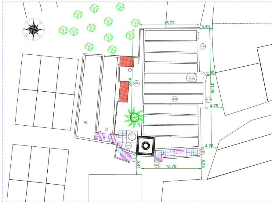
Fig. 3.7 - Plan de masse de la mosquée.
