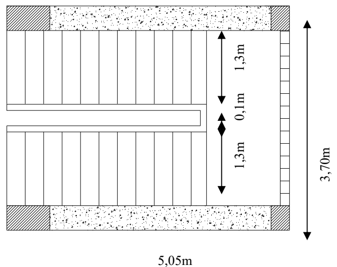
fig(V.2) Dessin en plan de l'escalier
