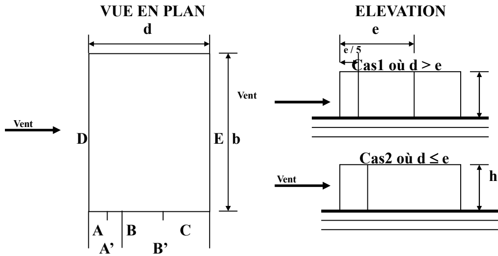
Fig.(VII.2) répartition des coefficients de pression (paroi verticale)
