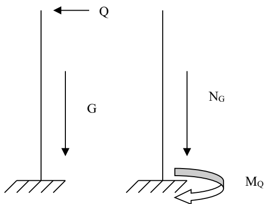
Schéma statique
