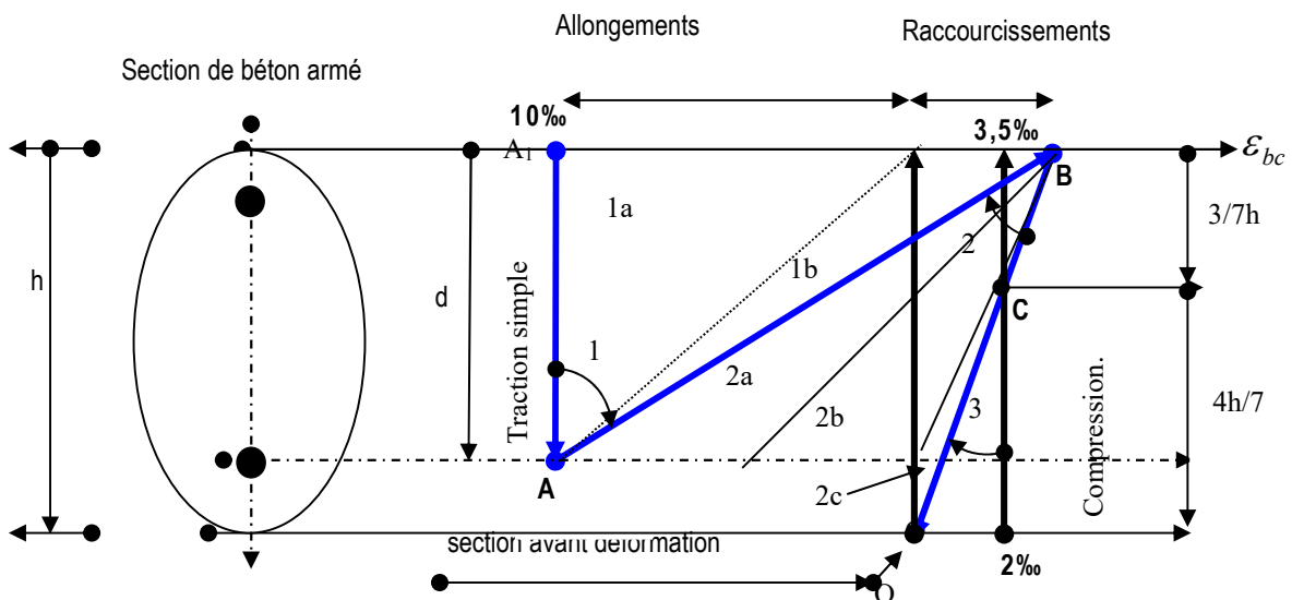
Fig (III.1) : Diagramme des déformations de la section (Règle des Pivots)
