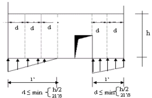
Figure (VII.2): Schéma de voile
