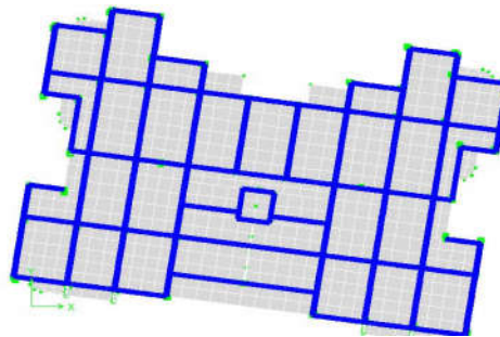
Mode3 : T = 0,566 s
