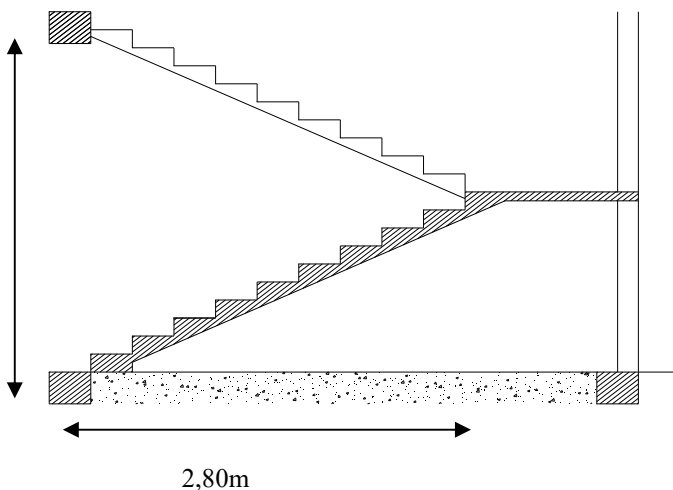
Fig (V.1) Dessin en elevation de l'escalier
