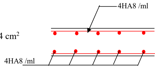
fig(V.6). Schéma de ferrailage de l'acrotère
