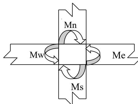
Figure VIII.1.10: Dimensionnement d'un noeud poutre - poteau
