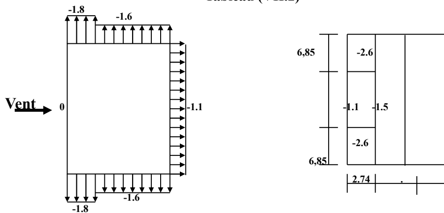
Fig (VII.4) répartitions des coefficients de pression
