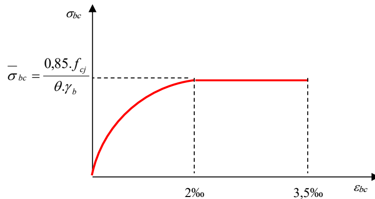
Fig. (III.2) : Diagramme parabole – rectangle (béton)
