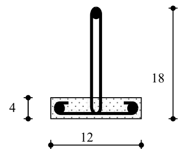
Figure (V.8) Poutrelle préfabriquée
