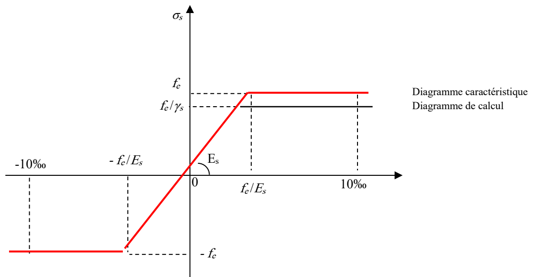
Fig. (III.3) : Diagramme contraintes déformations (Acier) pour HA1.3.et4 et rondes lisses \epsilon_s : Allongement relatif de l'acier, limité à 10 ‰.
