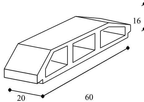
fig(V.7) : Corps Creux
