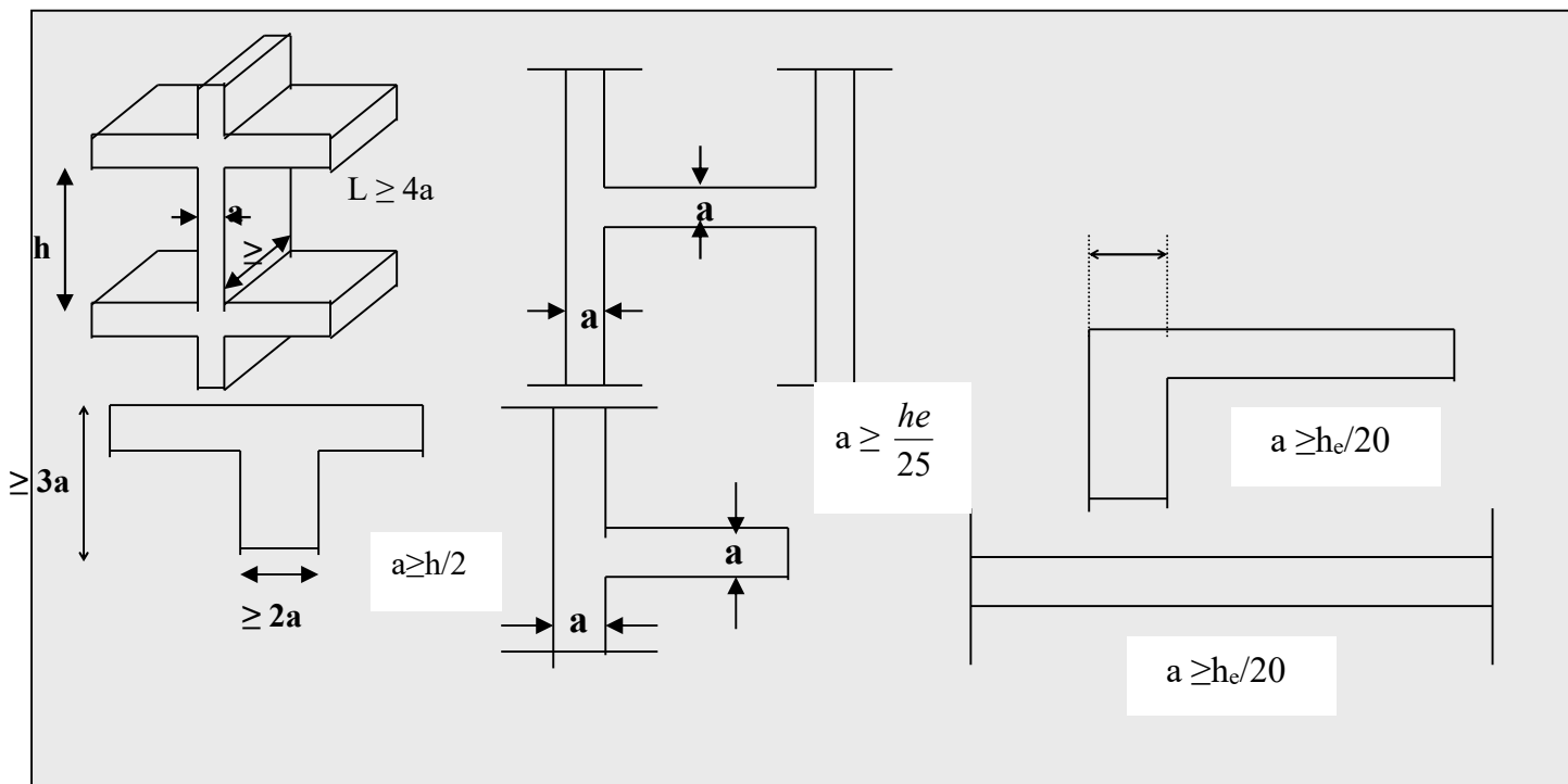
Fig.( IV.7) : Coupes de voiles
