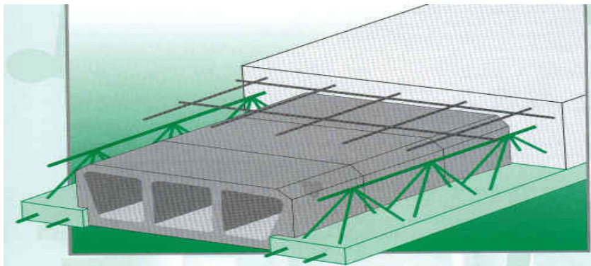
Fig.( IV .1) : Dessin d'un plancher en corps creux
