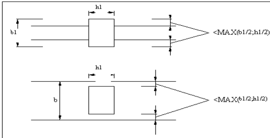
Figure.( IV.6 ) : Dimensions à respecter pour les poutres.
