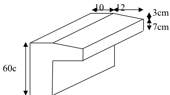
Fig.( IV.3 ) : Dessin de l'acrotère
