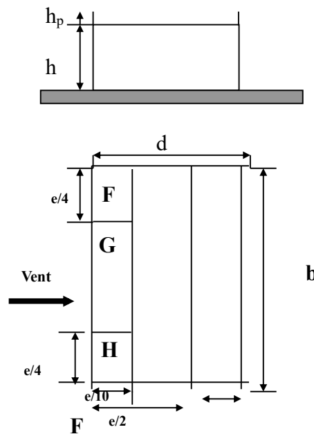
Fig.(VII.3) répartitions des coefficients de pression (Acrotère)
