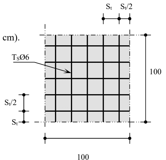
Fig. (V.10) Disposition constructive des armatures de la dalle de compression
