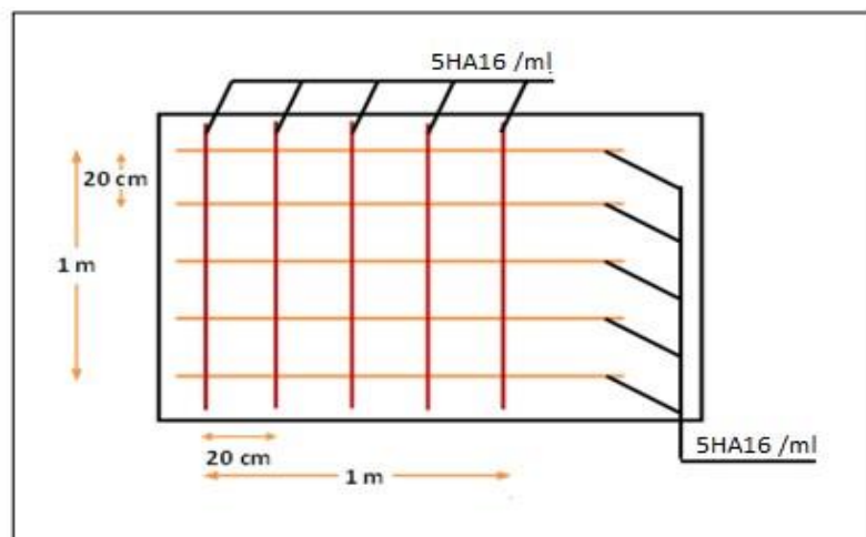
Figure 109.VII.:Ferrailage du mur de soutènement
