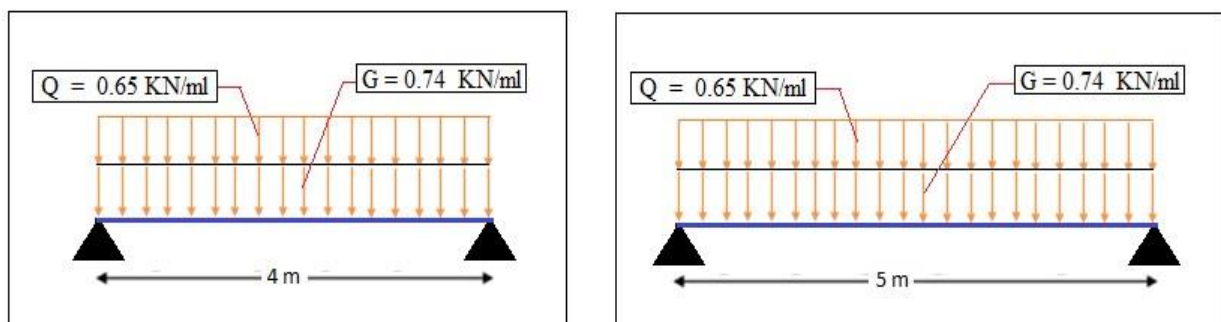
Figure 40.III.:Schéma des charges appliquées sur la poutrelle
