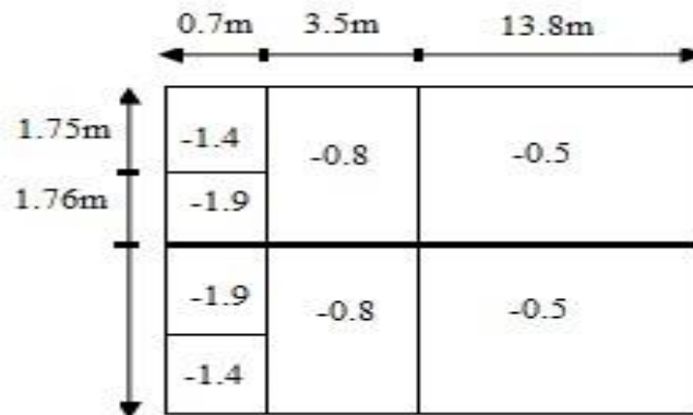
Figure 80.V.: Valeurs des pressions extérieures pour la toiture.
