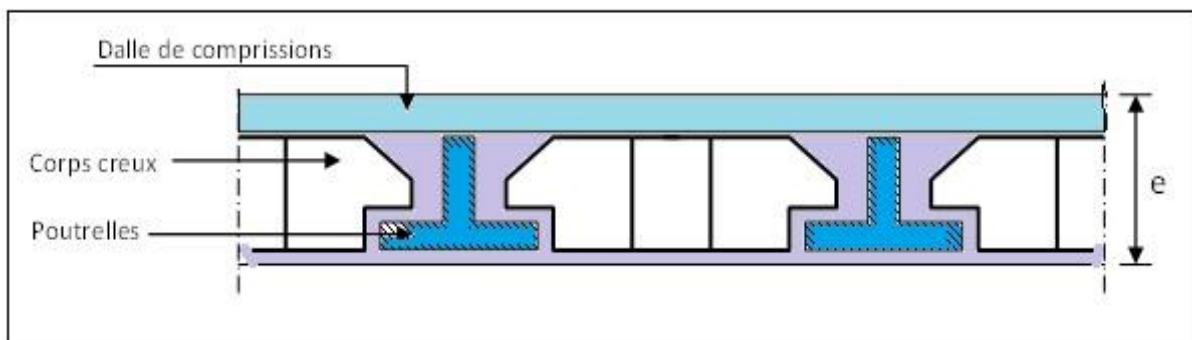
Figure 15.II. :Schéma d'une dalle à corps creux.
