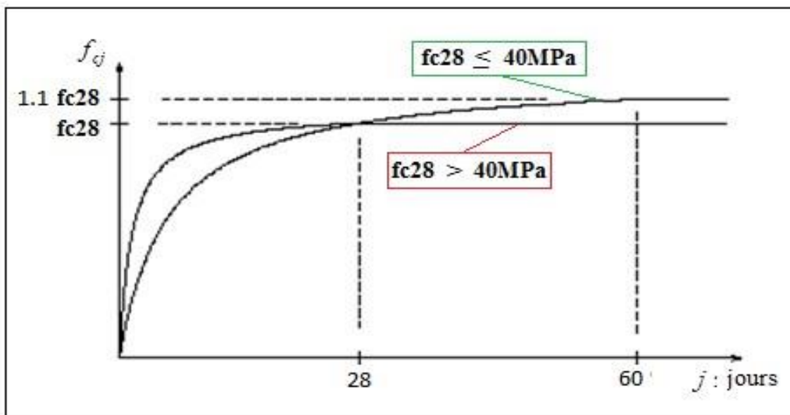
Figure 7.I.: Evolution de la résistance f_{cj} en fonction de l'âge du béton
