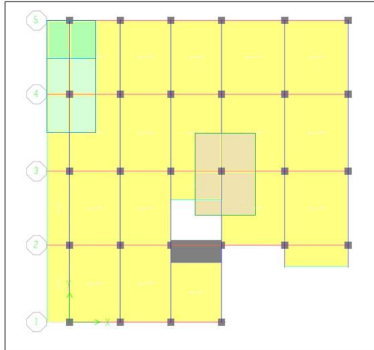
Figure 23.II.:choix des poteaux les plus sollicitent
