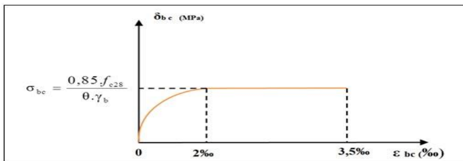
Figure 10.I. : Diag Contraintes – Déformations du béton à l'ELU (parabole rectangle)
