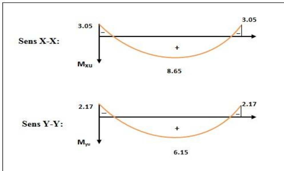
Figure 33.III.:Diagrammes des moments à L'ELS.
