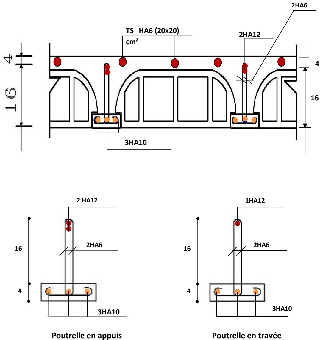
Figure 54. III.: Schéma de ferrailage du plancher (sens x-x)
