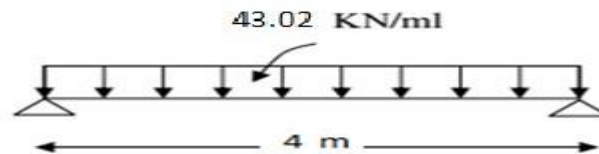
Figure 64.III. : Schéma statique de poutre palier (escalier type 02)
