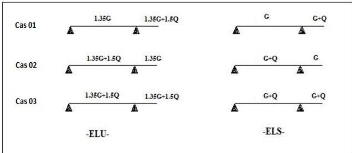
Figure 59.III.: Combinaison des charges selon chaque cas
