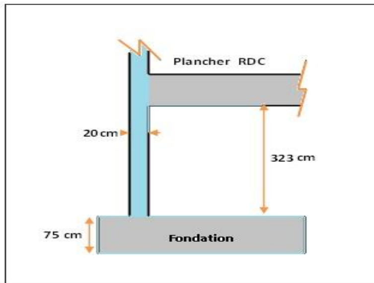
Figure 105.VII.: Schéma du voile périphérique
