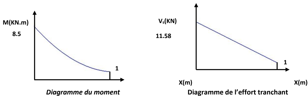
Figure 28.III.:Diagramme des sollicitations à l'ELU
