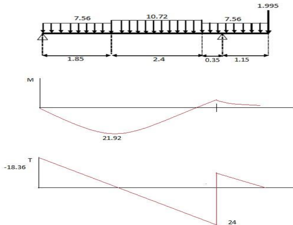
Figure 61. III.: Le schéma statique à L'ELS (escalier type 01)
