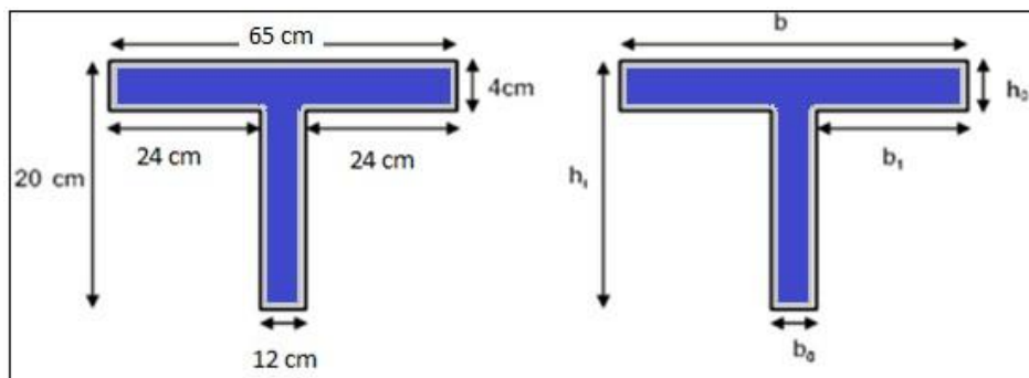
Figure 38.III.:Schéma d'une poutrelle
