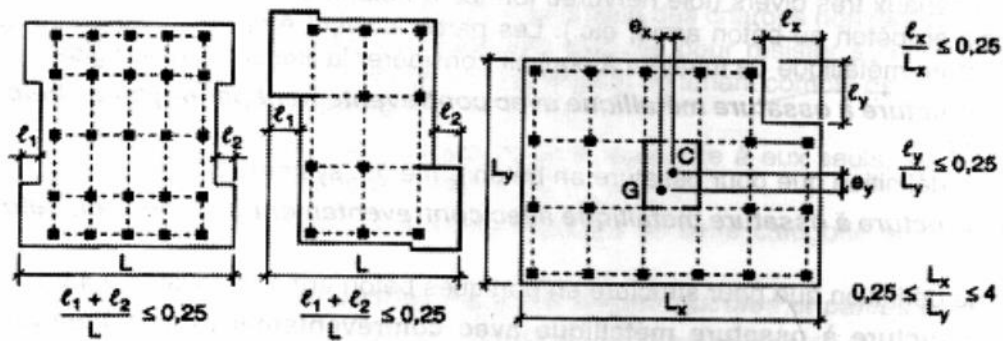
Figure 66.IV. : Limites des décrochements en plan.
