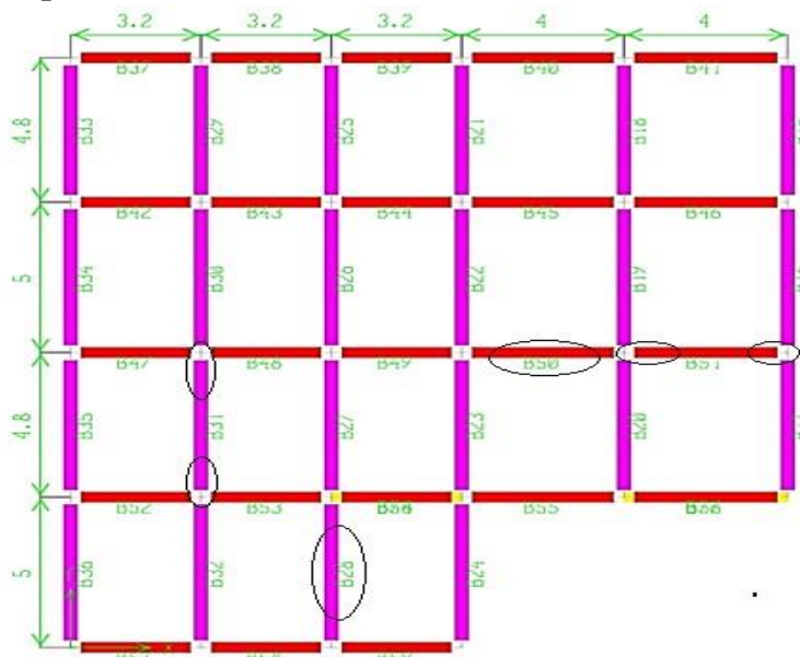
Figure 88.VI.: Identification des poutres (les plus sollicitées).
