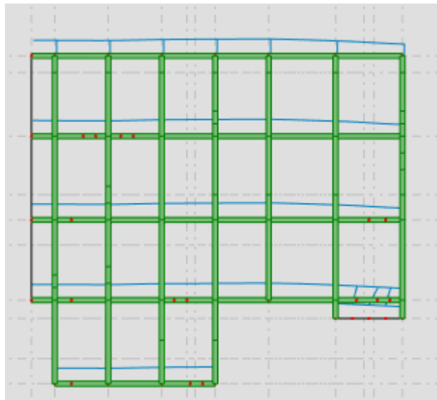
Figure 70.IV: LE 2 ème mode de déformation de la structure à cause des efforts sismiques 3D translation suivant l'axe YY' (résultats de l'RSA 2019).
