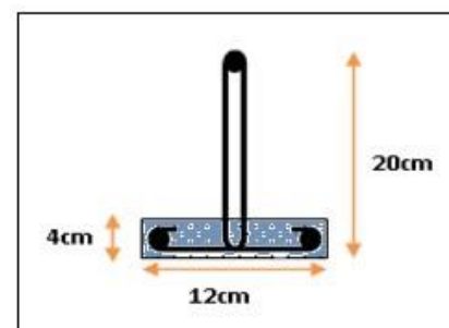
Figure 39.III.: Schéma de la nervure
