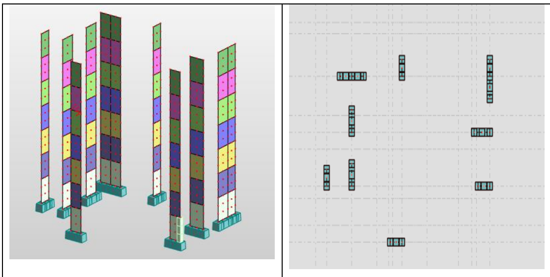
Figure 68.IV. : La disposition des murs voile (variante 1).
