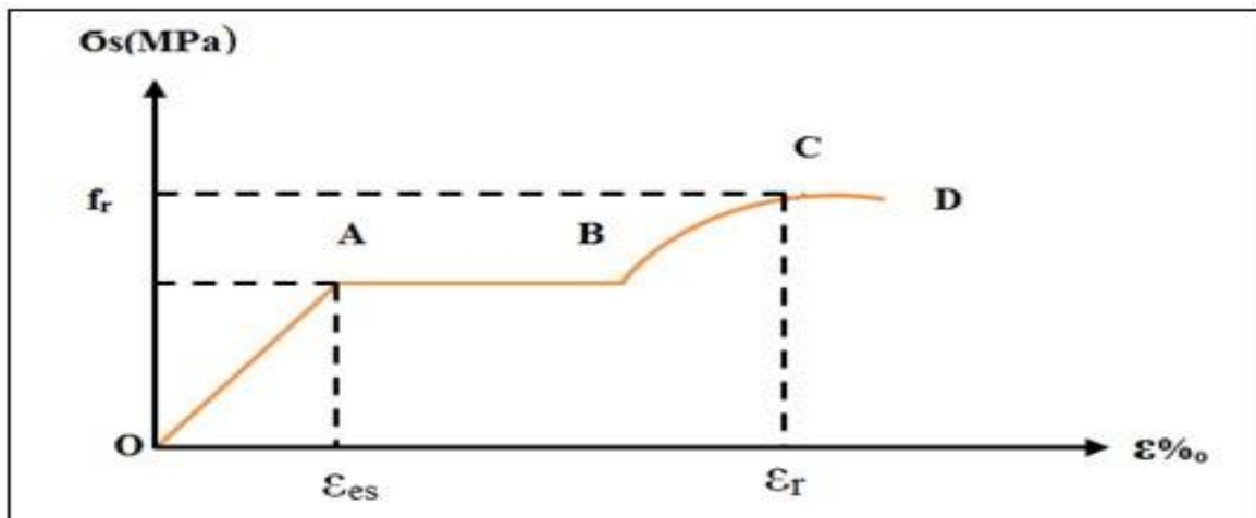
Figure 13.I. :Diagramme contrainte déformation de l'acier
