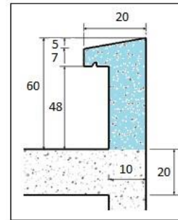
Figure 17 II.3 Schéma d'une Acrotère
