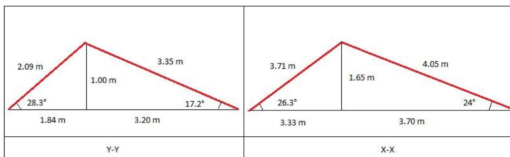
Figure 83.V.: Schémas de la toiture
