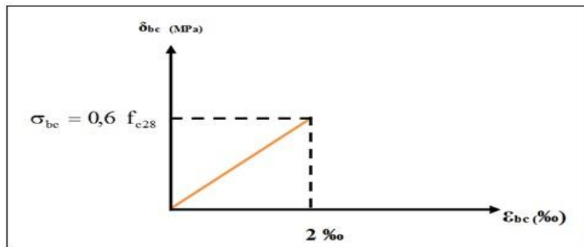
Figure 12.I.: Diagramme Contraintes Déformations du béton à l'ELS
