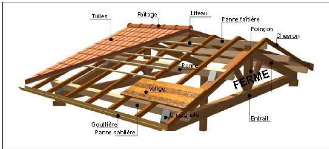
Figure 84.V.: Composants d’une toiture
