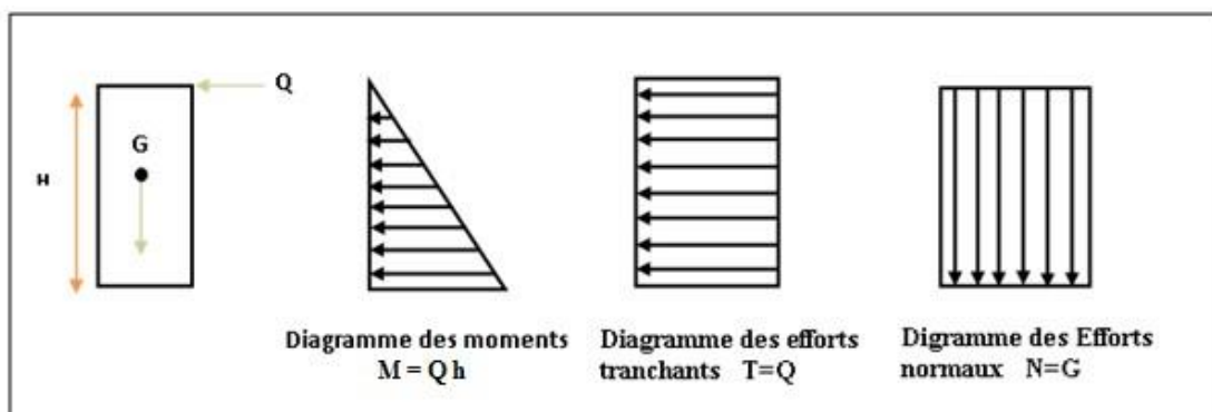
Figure 25.III.: Schéma statique de l'acrotère
