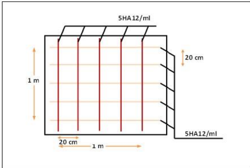
Figure 106.VII.: Schéma de ferrailage du voile périphérique
