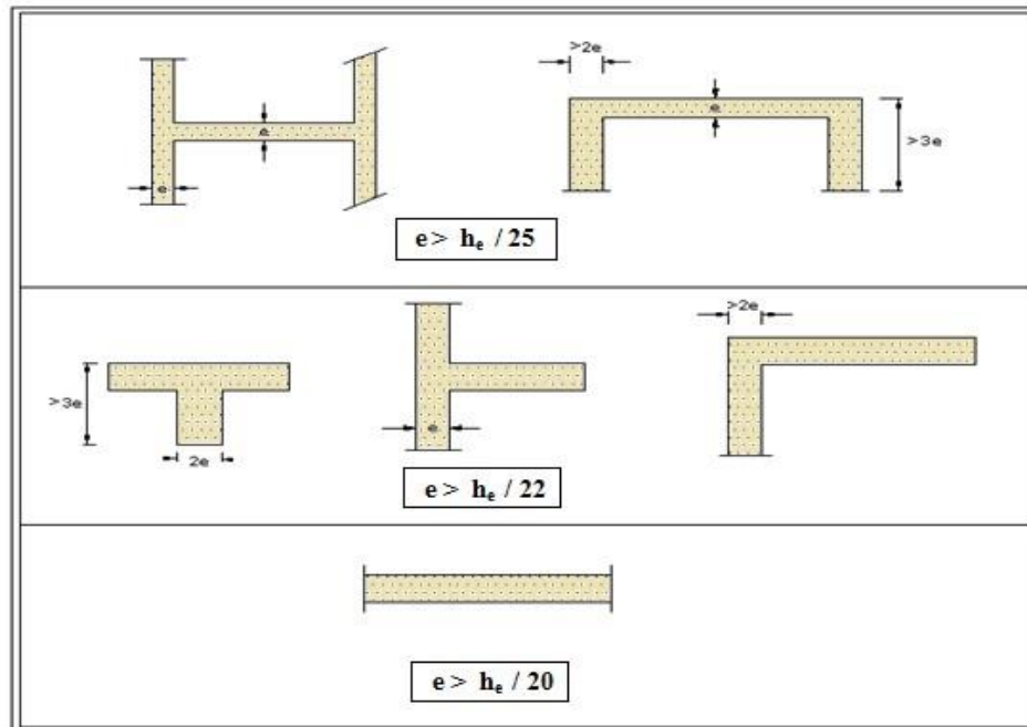
Figure 22.II.:Coupe de voile en plan.
