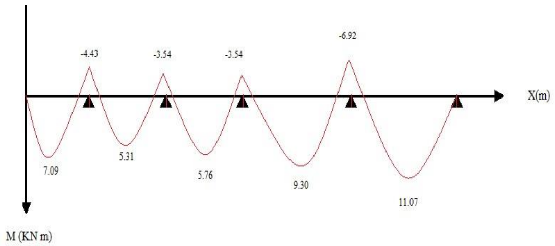
Figure 46.III.: Diagramme des moments à l'ELU (Poutrelle a 5 travées).
