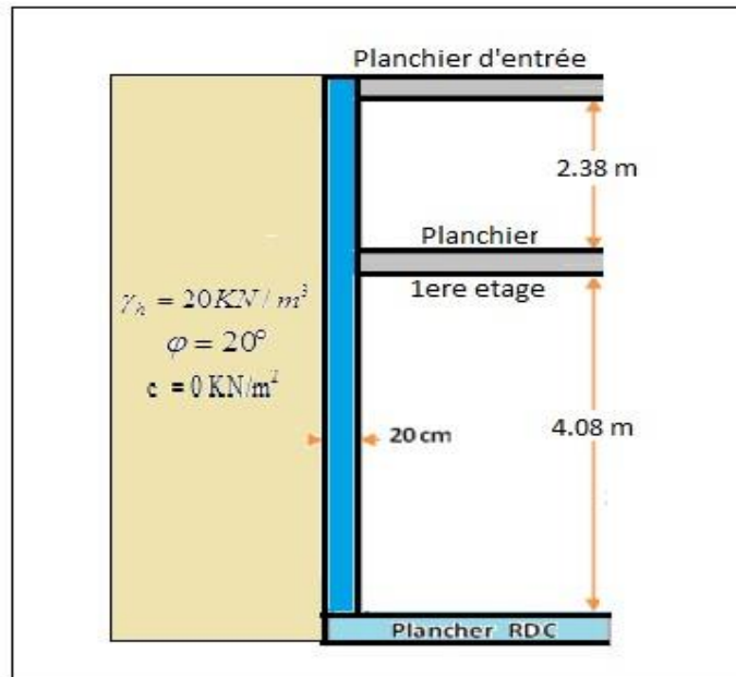
Figure 107.VII.: Mur de soutènement en contact avec le sol
