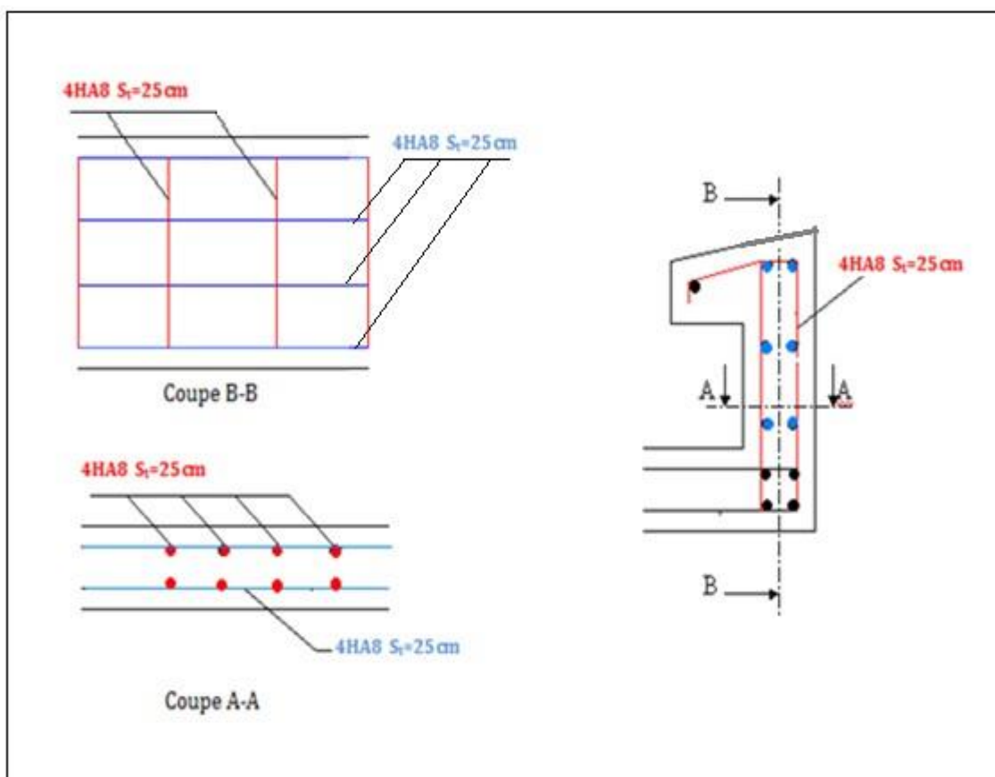
Figure 26.III.: Schéma de ferrailage de l'acrotère
