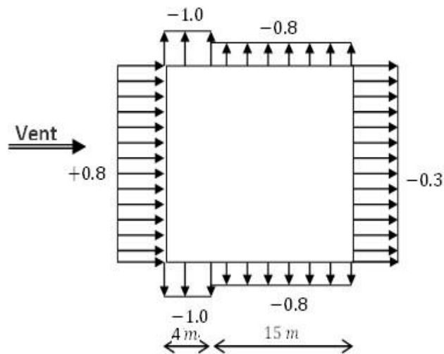
Figure 76. V.: Valeurs des pressions extérieures pour les parois verticales.
