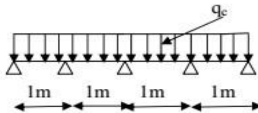
Figure 87.V.: Schémas de chargement de chevron
