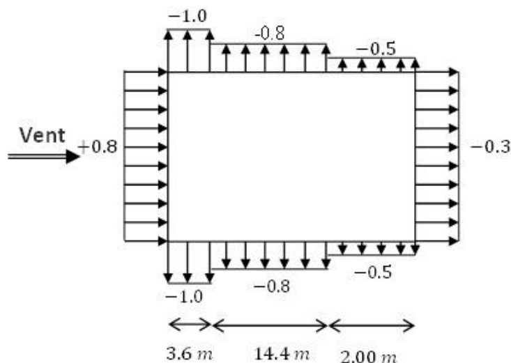
Figure 77.V.: Valeurs des pressions extérieures pour les parois verticales.
