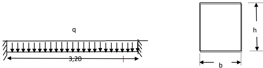
Figure 62.III.: Schéma Statique de la poutre palière (escalier type 01) La poutre palière se calcul a ELU puisque la fissuration est considéré peu nuisible.
