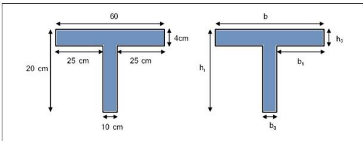
Figure 16.II.: Schéma d'une poutrelle
