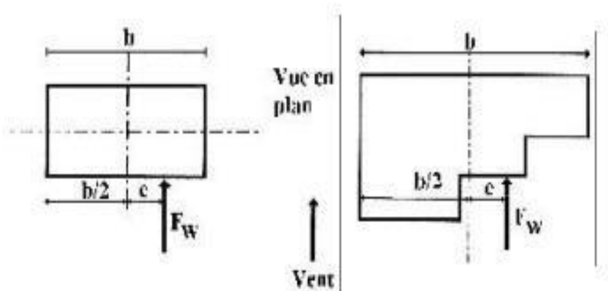
Figure 82.V.: Excentricité de la force globale
