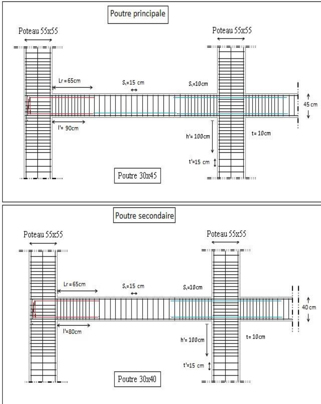
Figure 90.VI.: Disposition constructif en RDC
