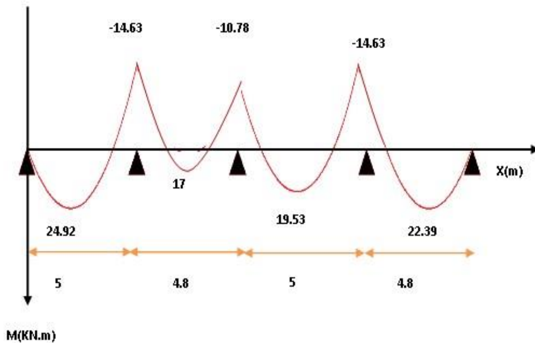
Figure 50.III.: Diagramme des moments à l'ELU (Poutrelle a 4 travées).
