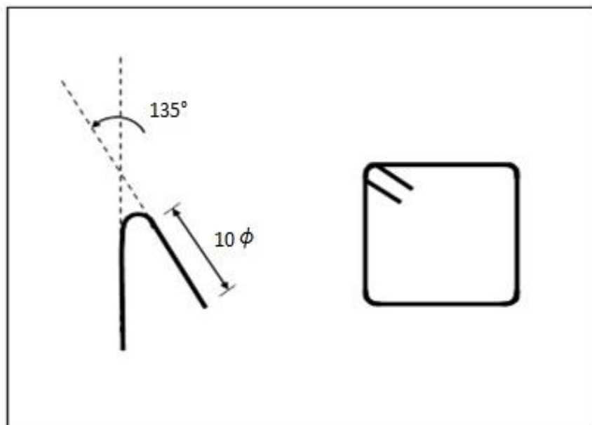
Figure 95 .VI.: Détail des armatures transversales
