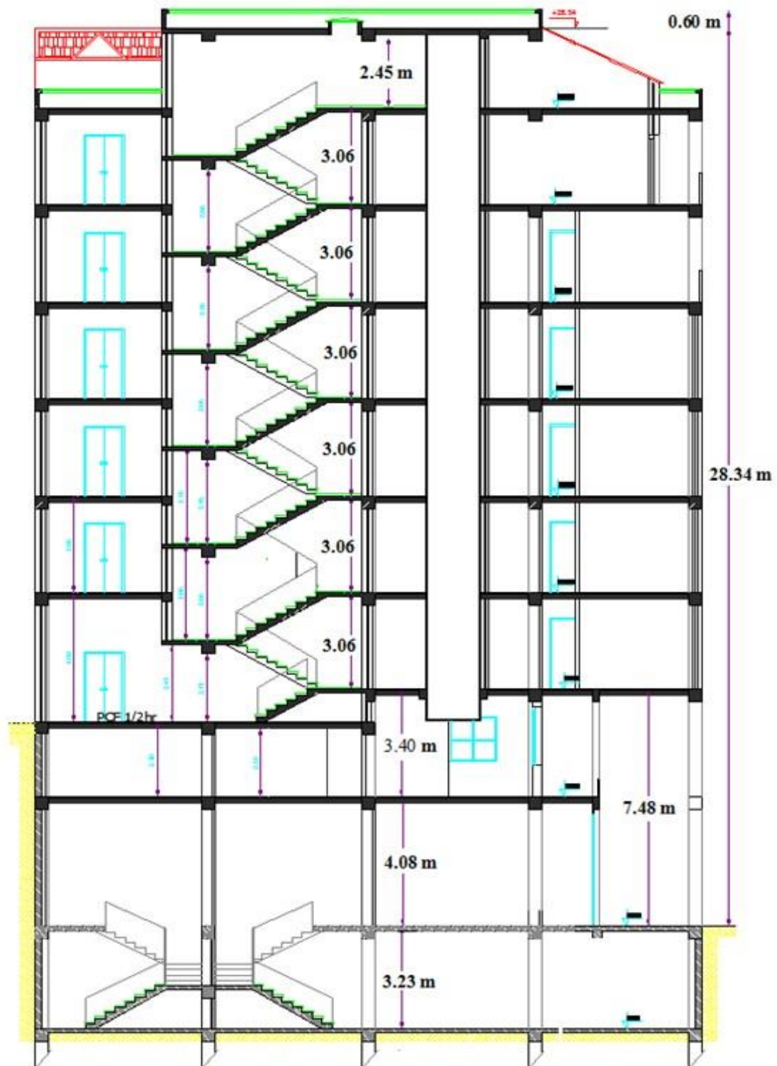
Figure 2. I.: Coupe verticale A-A de la structure
