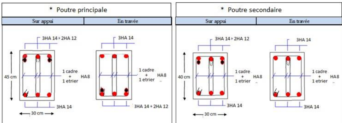
Figure 89.VI.: Schémas de ferrailage des poutres par zone
