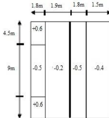
Figure 79.V. : Valeurs des pressions extérieures pour la toiture.
