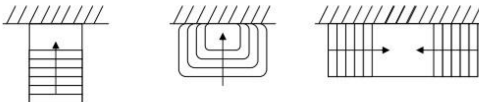
Figure 58.III.: Les systèmes les plus courants pour les escaliers extérieurs.
