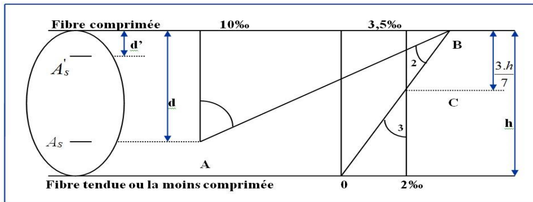
Figure 9.I.: Diagramme des déformations limites de la section
