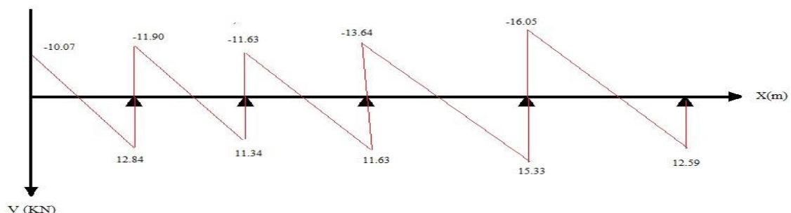
Figure 45.III.: Diagramme des efforts tranchants à L'ELU (Poutrelle a 5 travées).
