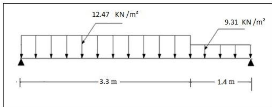
Figure 63.III.: Schéma statique à L'ELU et à L'ELUS (escalier type 02)
