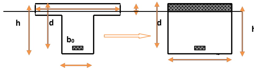
Figure 53.III.: Coupe de Section Rectangulaire et Section en T
