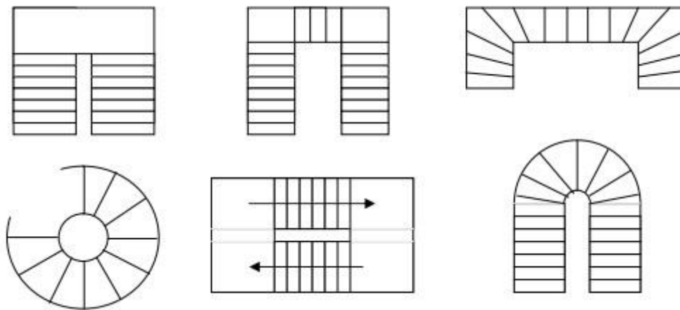
Figure 57.III.: Les systèmes les plus courants pour les escaliers intérieurs.
