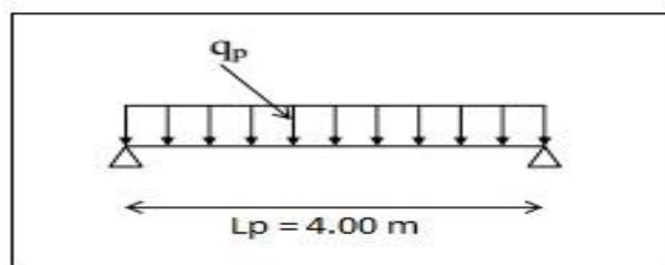
Figure 85.V.: Schémas de chargement de panne dans les deux sens
