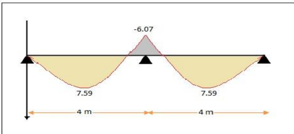
Figure 44. III.:Diagramme des moments à L'ELS (Poutrelle a 2 travées).
