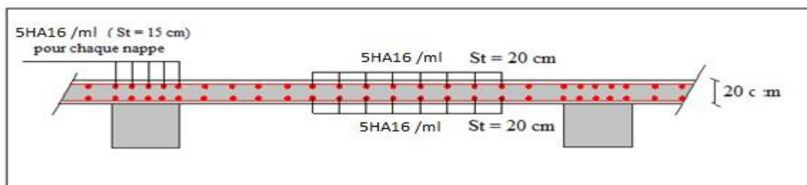
Figure 110.VII.:Ferrailage du mur de soutènement (Coupe transversale)
