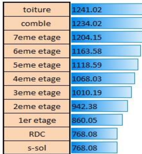
Figure 74.V.: Répartition de la pression dynamique
