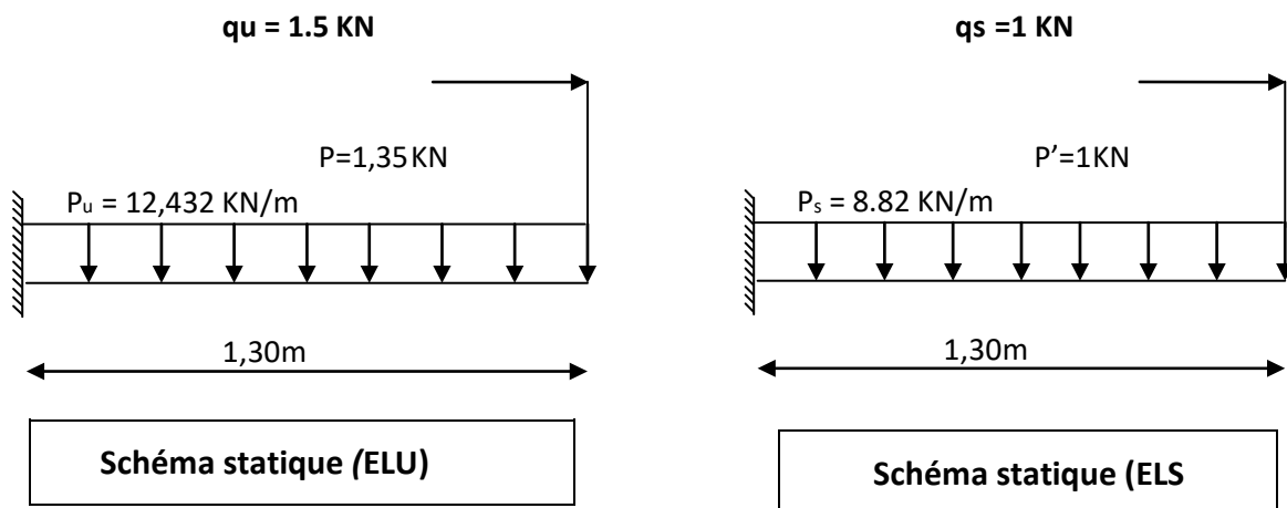
Figure 27.III. : Schéma statique pour calcul du balcon a l'ELU et a l'ELS
