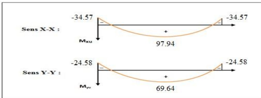
Figure 102.VII.: Diagrammes des moments à L'ELS (Radier).
