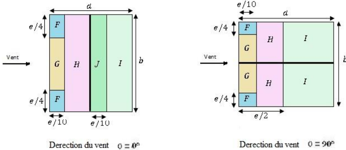
Figure 78.V.: Légende pour la toiture.
