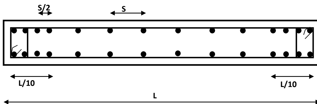
Figure 91.VI.: Disposition des armatures verticales dans le voile.
