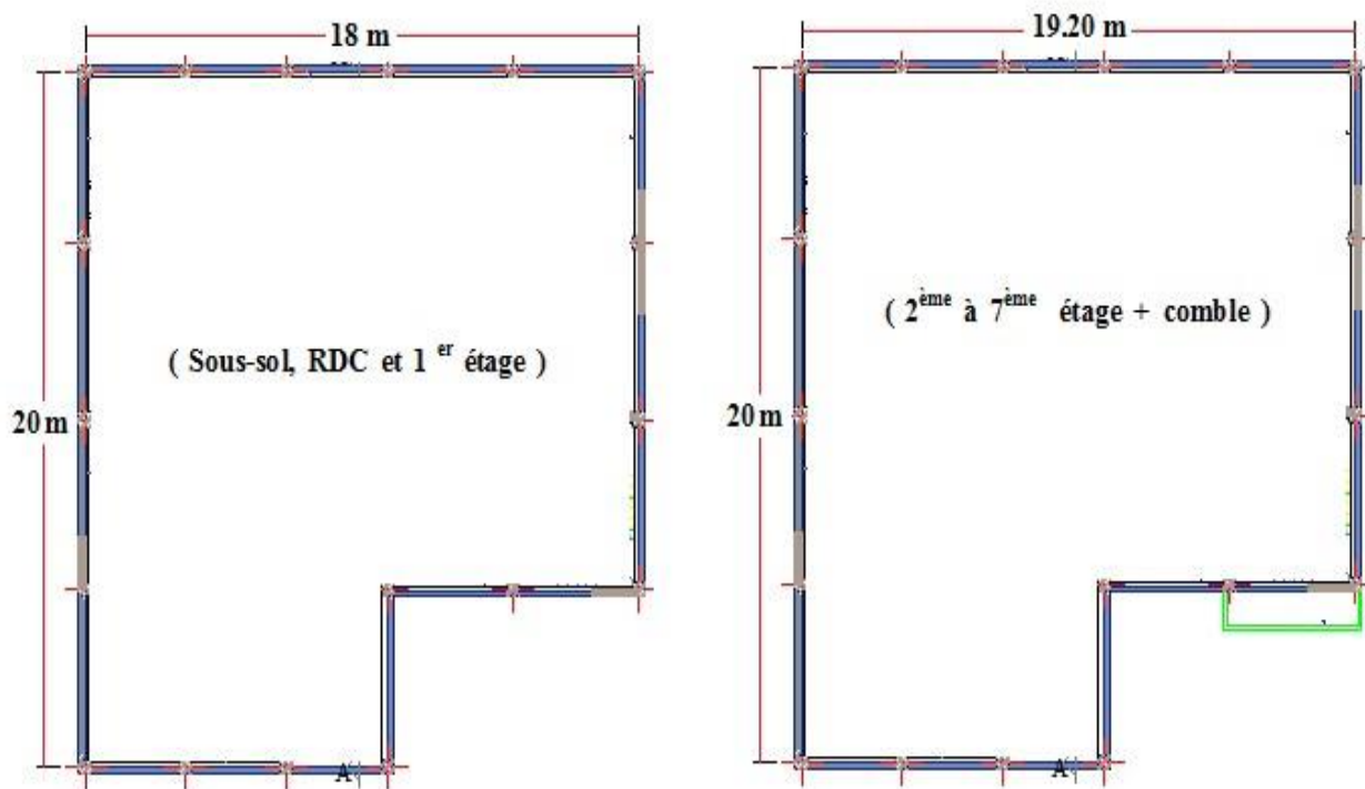
Figure 1.I: Vue en plan de la structure 1
