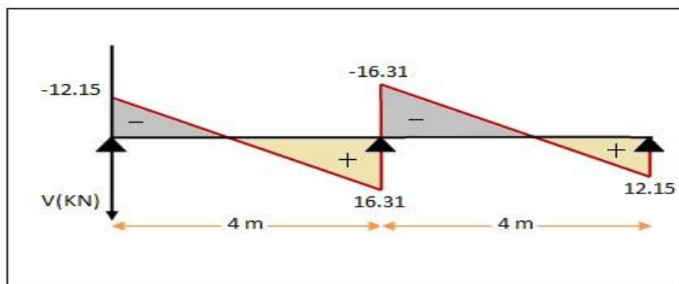
Figure 41.III.:Diagramme de l'effort tranchant à L'ELU (Poutrelle a 2 travées).
