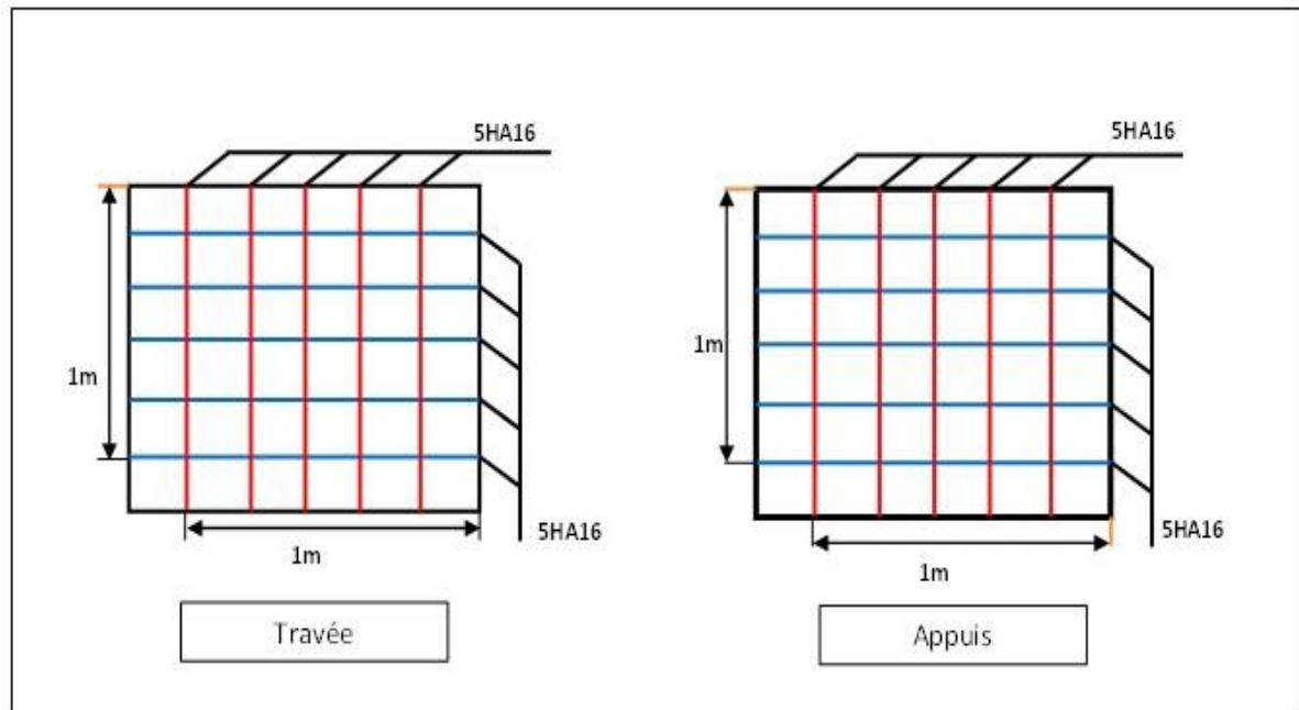
Figure 104.VII.: Schéma de ferrailage du radier
