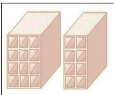
Figure 4.I: Brique creuse
