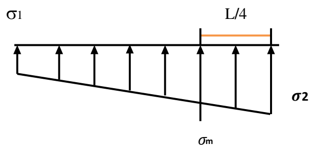
Figure 99.VII.:Diagramme des contraintes
