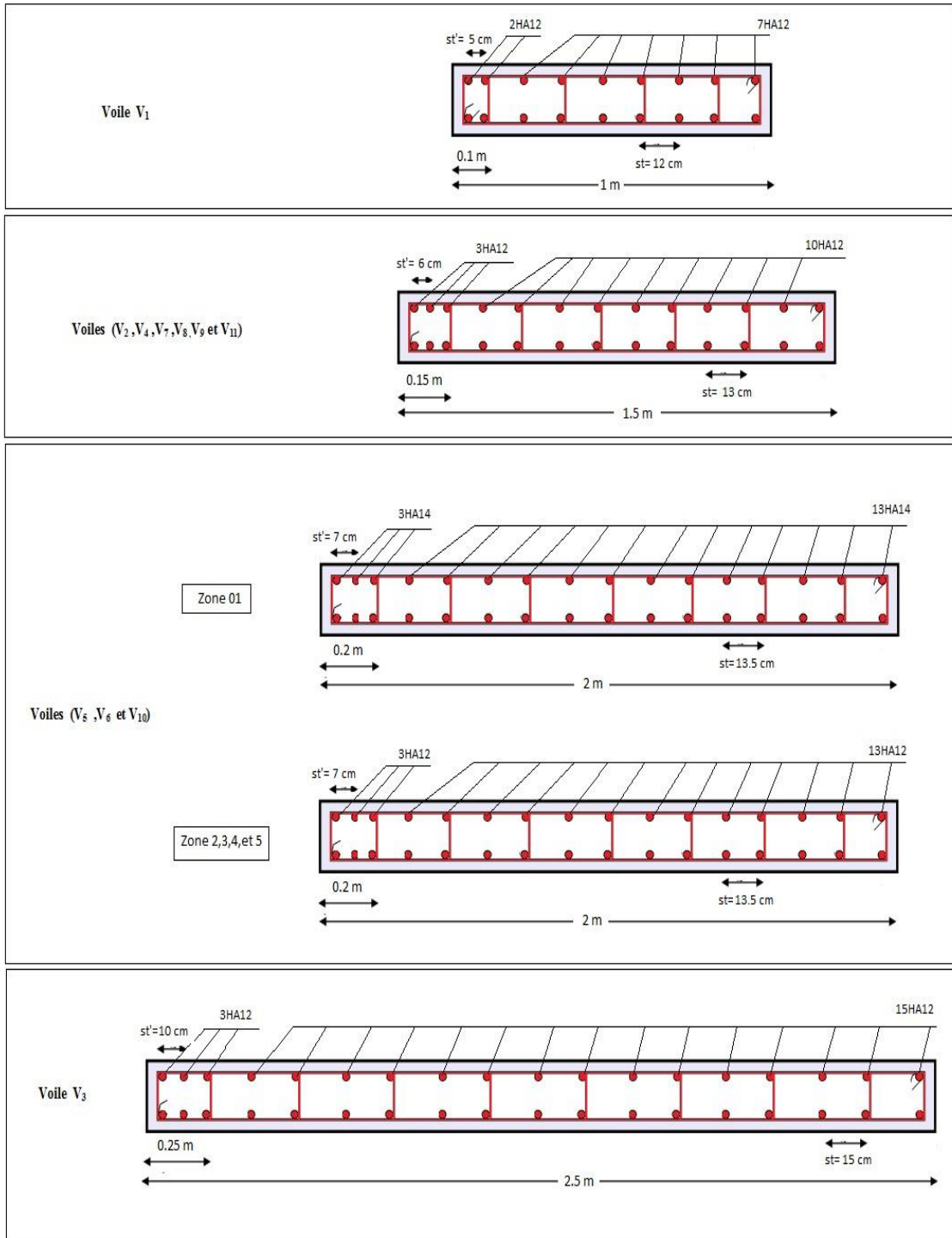
Figure 93.VI.: Schémas de ferrailage des voiles
