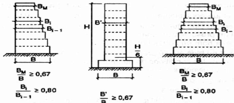
Figure 67.IV. : Limite des décrochements en élévation.
