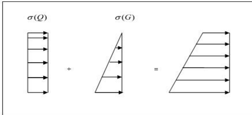
Figure 108.VII.: Répartition des contraintes sur le mur de soutènement
