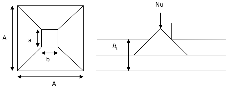
Figure 98.VII.: Présentation de zone d'impact de la charge compactée
