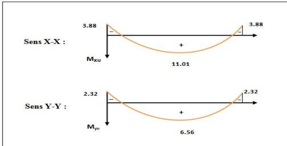
Figure 32.III.:Diagrammes des moments à L'ELU.
