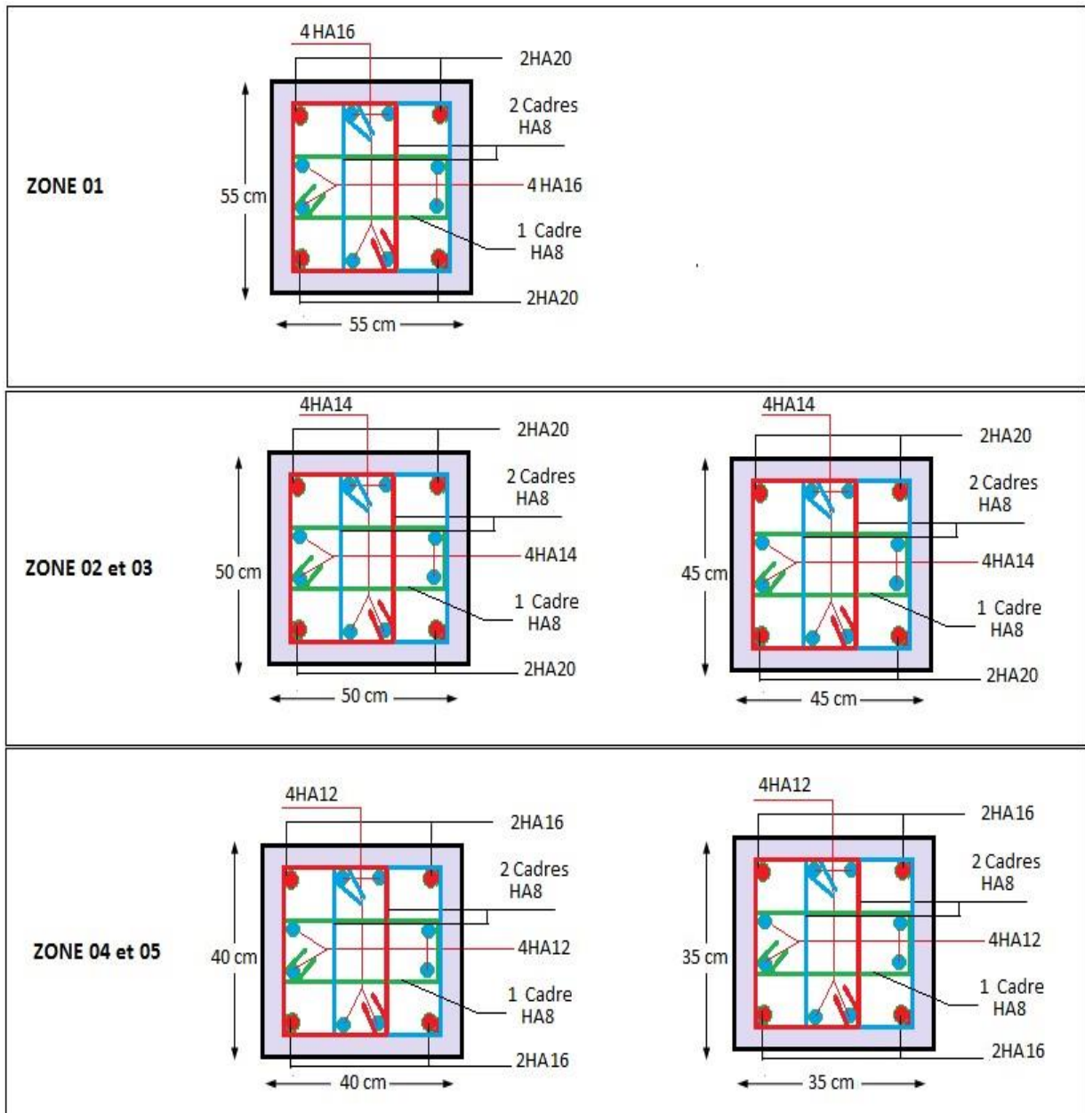
Figure 96.VI.: Schéma de ferrailage des poteaux
