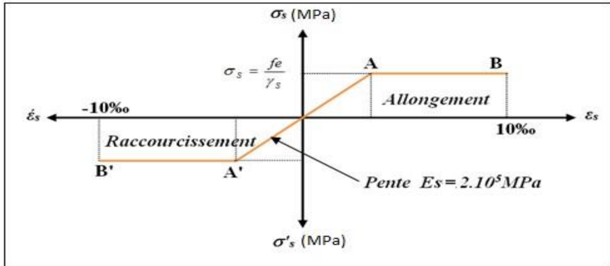
Figure 14.I.: Diagramme contraintes- déformations de calcul
