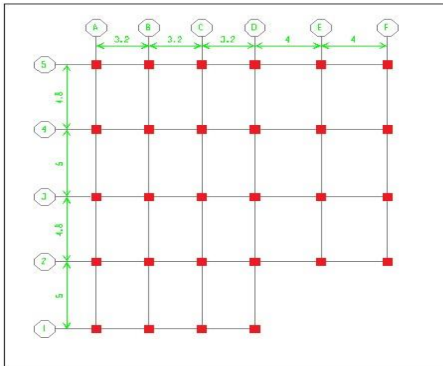
Figure 97.VII.:Dispositions des semelles
