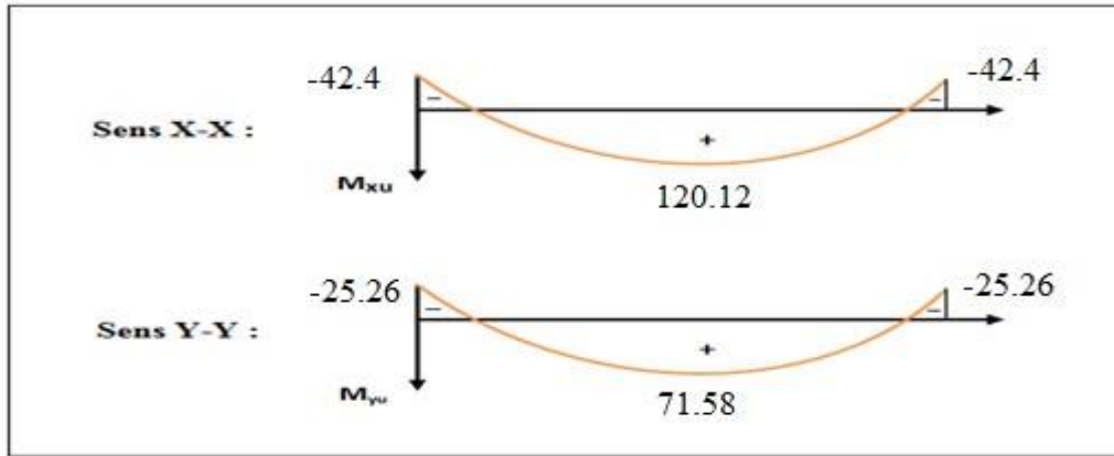
Figure 101.VII.: Diagrammes des moments à L'ELU (Radier).
