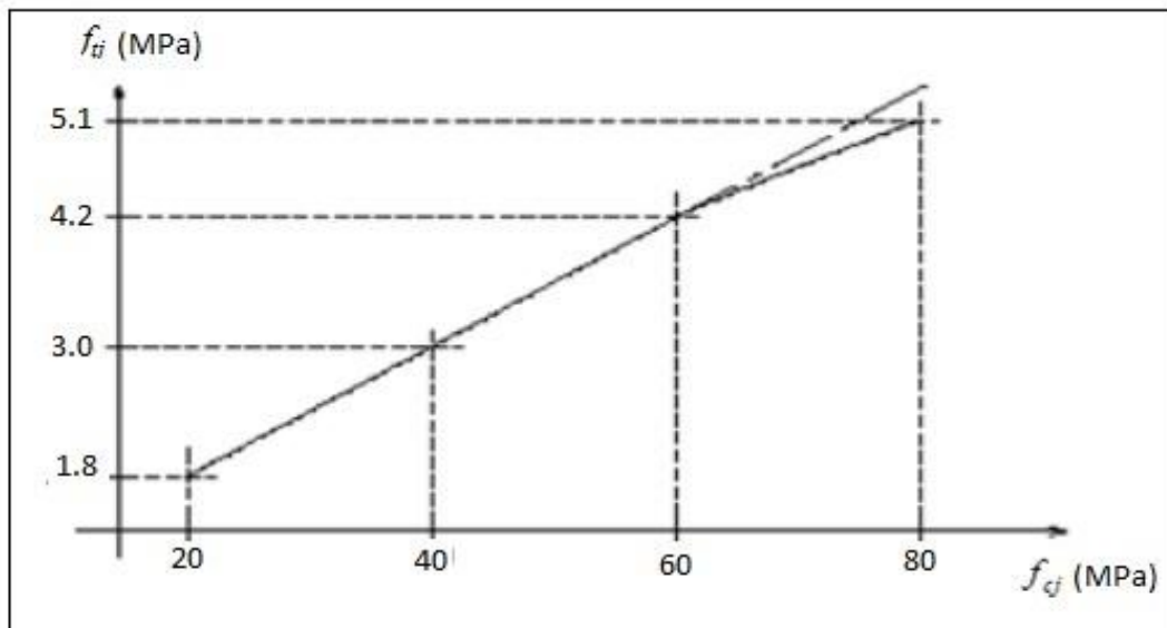
Figure 8.I. : Evolution de la résistance à la traction f_{tj} en fonction de f_{cj}
