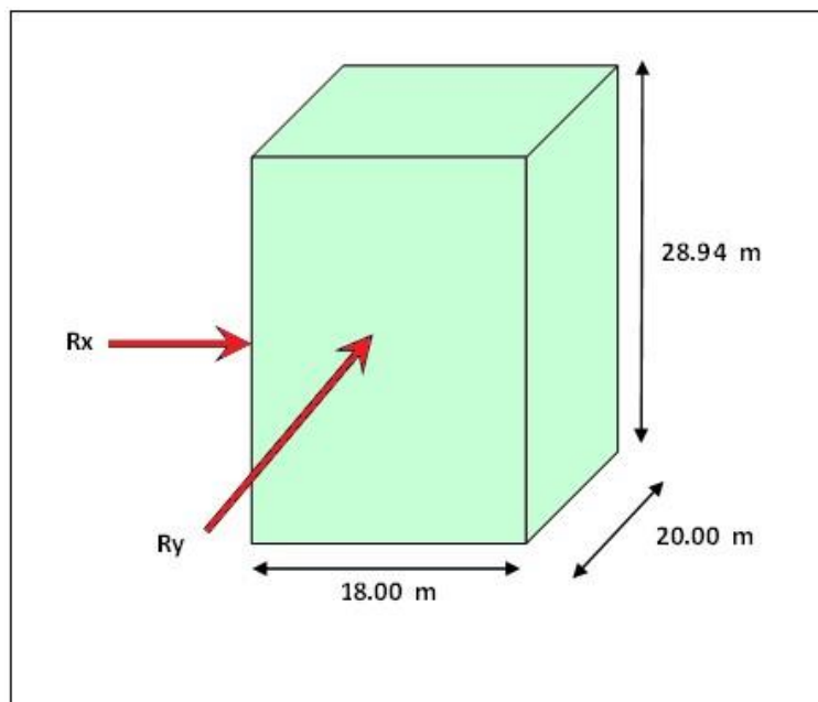
Figure 73. V.: Action du vent sur la structure
