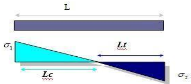
Figure 92.VI.:Diagramme des contraintes
