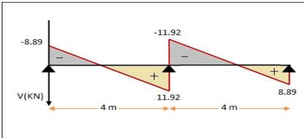
Figure 43.III.:Diagramme de l'effort tranchant à L'ELS (Poutrelle a 2 travées).
