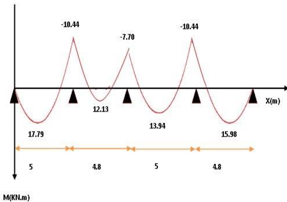
Figure 52. III.:Diagramme des moments à L 'ELS (Poutrelle a 4 travées).
