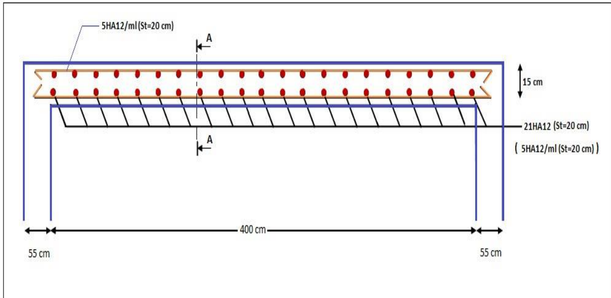
Figure 34.III.: Schéma de ferrailage de la dalle pleine
