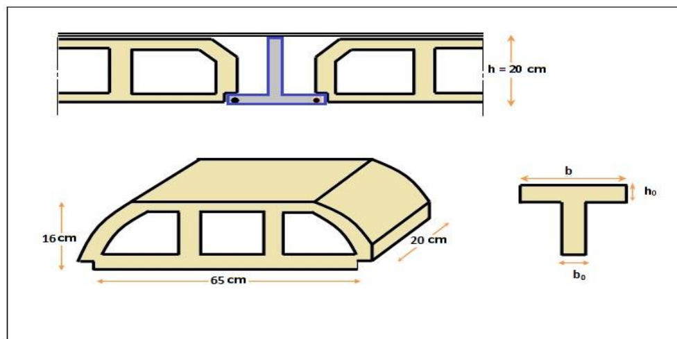
Figure 36.III.: Schéma coupe verticale de plancher
