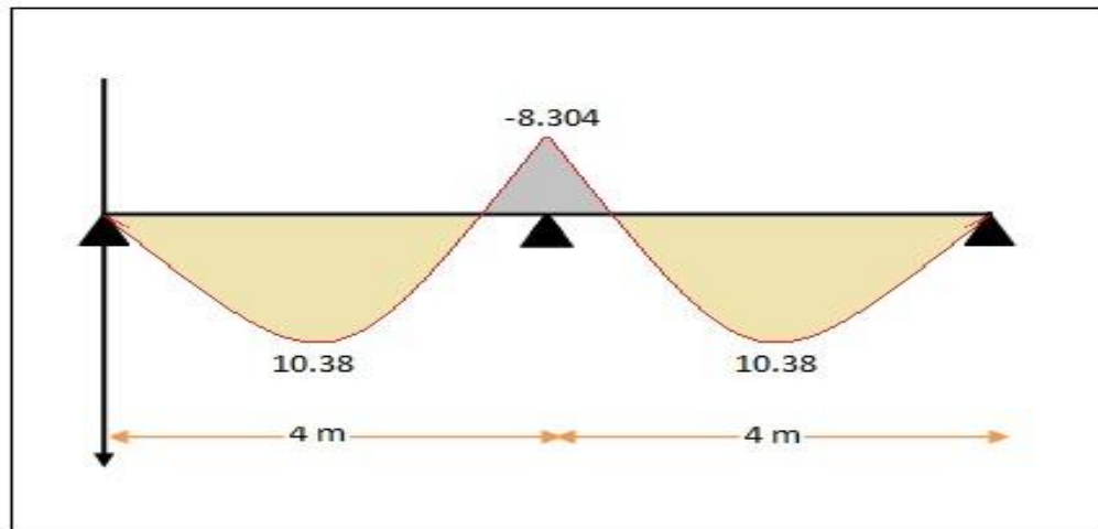
Figure 42.III.:Diagramme des moments à L'ELU (Poutrelle a 2 travées).
