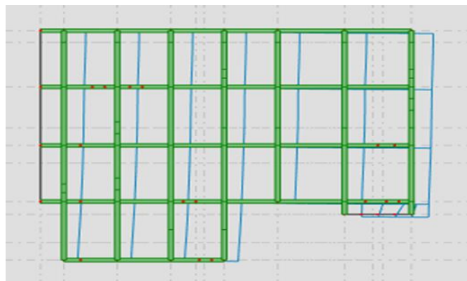
Figure 69.IV. : Le 1er mode de déformation de structure à cause des efforts sismiques 3D translation suivant l'axe XX' (résultats de l’RSA 2019).
