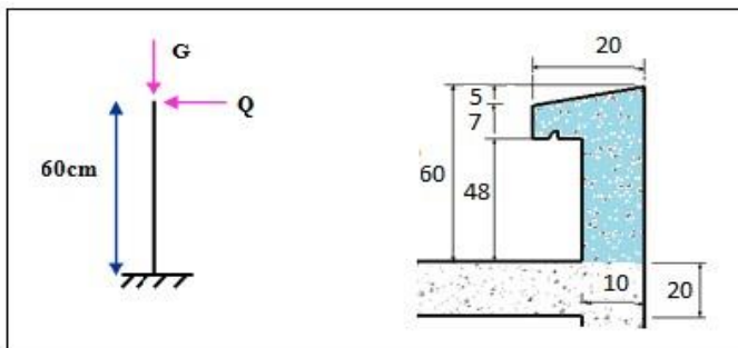
Figure 24.III.: Coupe verticale de l'acrotère
