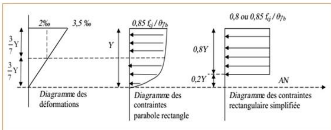
Figure 11.I.: Diagramme rectangulaire simplifié
