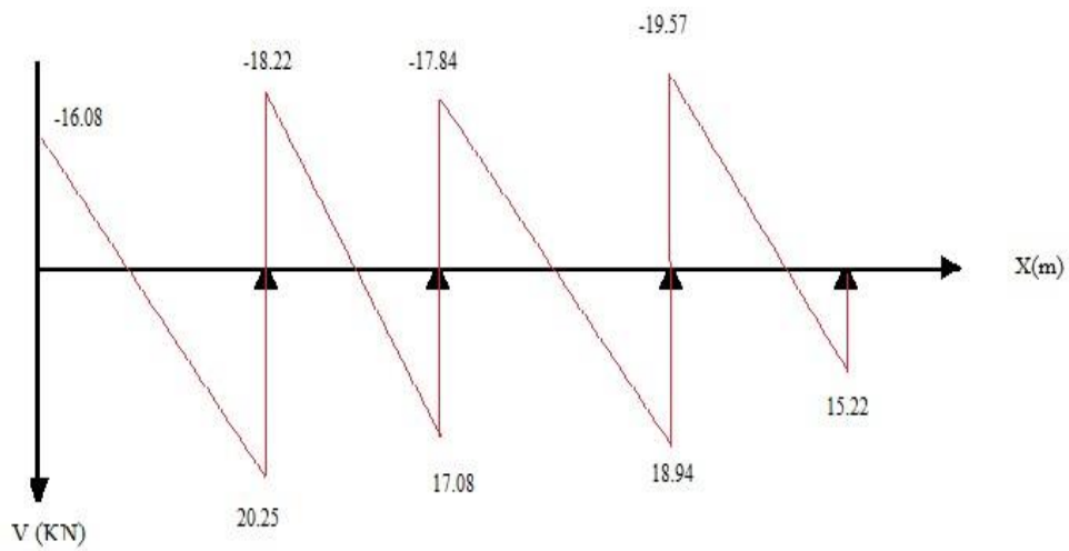
Figure 51.III.:Diagramme des efforts tranchants à L 'ELS (Poutrelle a 4 travées).
