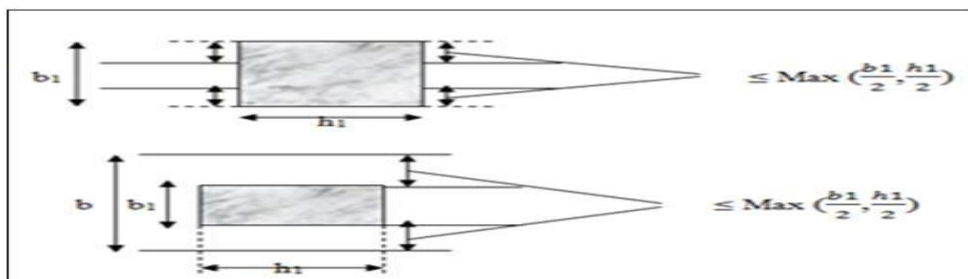
Figure 18.II.: Dimensions à respecter pour les poutres
