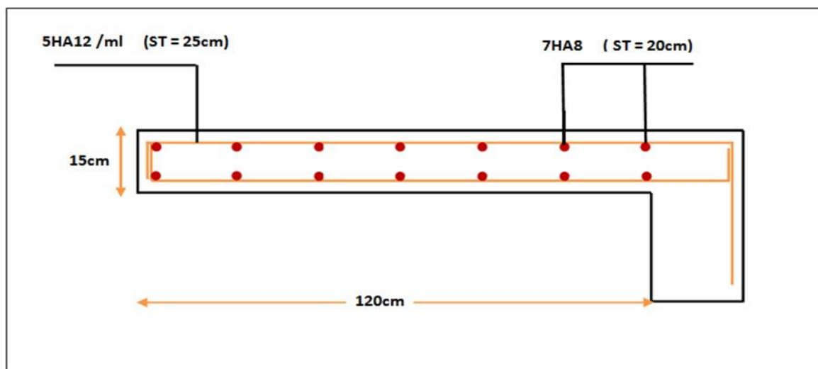
Figure 30.III.: Schéma de ferrailage de balcon
