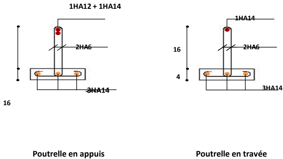
Figure 55. III: Schéma de ferrailage du plancher (sens y-y)
