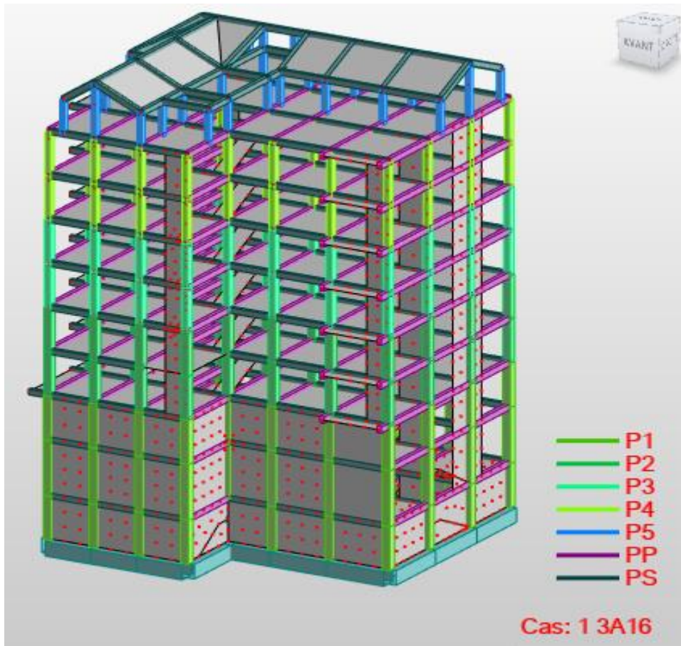
Figure 65.IV.: Vue de la structure en 3D
