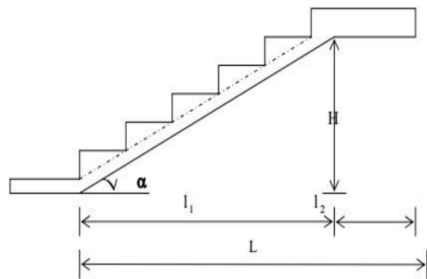
Figure 56.III.: Schémas d'un escalier
