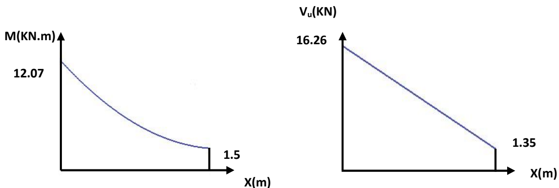
Figure 28.III.:Diagramme des sollicitations à l'ELU
