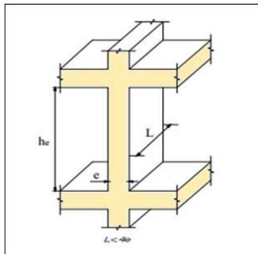
Figure 21.II.: Coupe de voile en élévation
