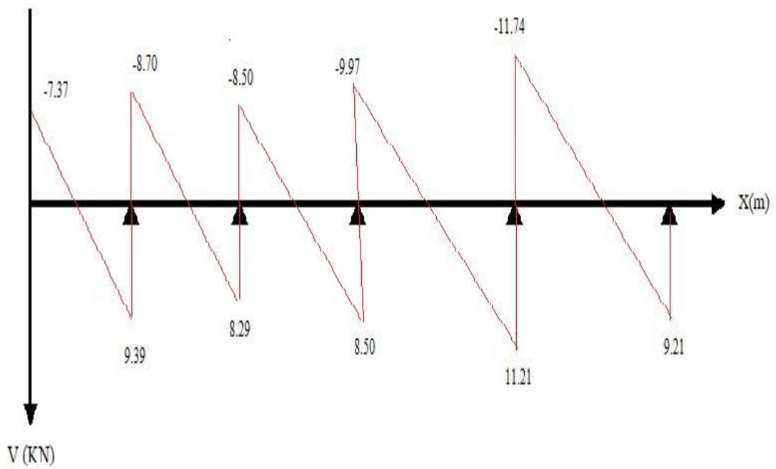
Figure 47.III.: Diagramme des efforts tranchants à L'ELS (Poutrelle a 5 travées).
