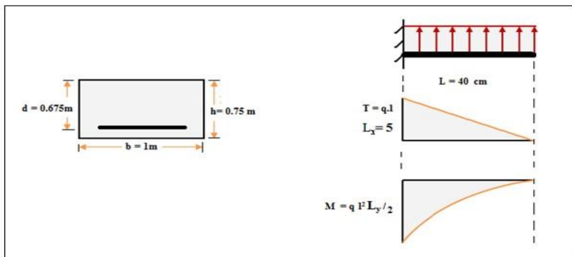
Figure 103.VII.: Schéma statique du débord
