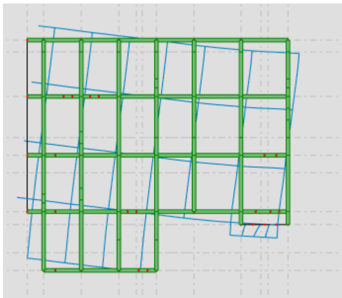
Figure 71.IV. : Le 3 ème mode de déformation de la structure à cause des efforts sismiques vue X-Y: torsion (résultats de l'RSA 2019).
