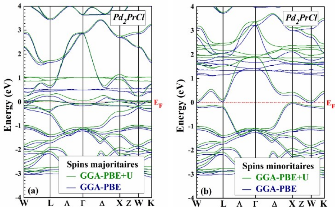
Figure III.3: Calcul spin-polarisé (SP) de la structure de bande du Pd 2 PrCl (a) spin majoritaires, et (b) spin minoritaires. La ligne horizontale montre l'énergie de Fermi.
