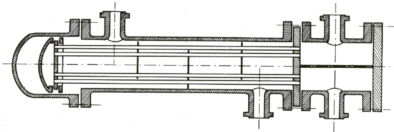
Figure II.2 Échangeur à faisceau constitué par des tubes en U
