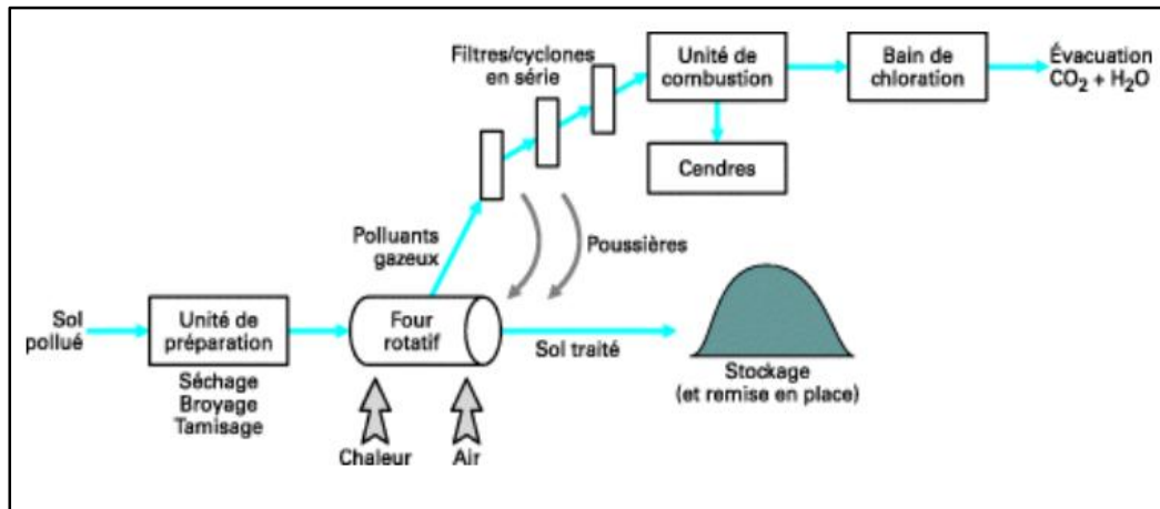
Figure. II.12. Schéma descriptif de l'incinération par four rotatif (Roudier, 2005 ; Dufresne, 2013)
