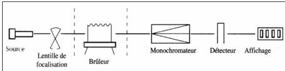
Figure IV.16. Schéma explicatif d'un spectrophotomètre (Mun, 2007)
