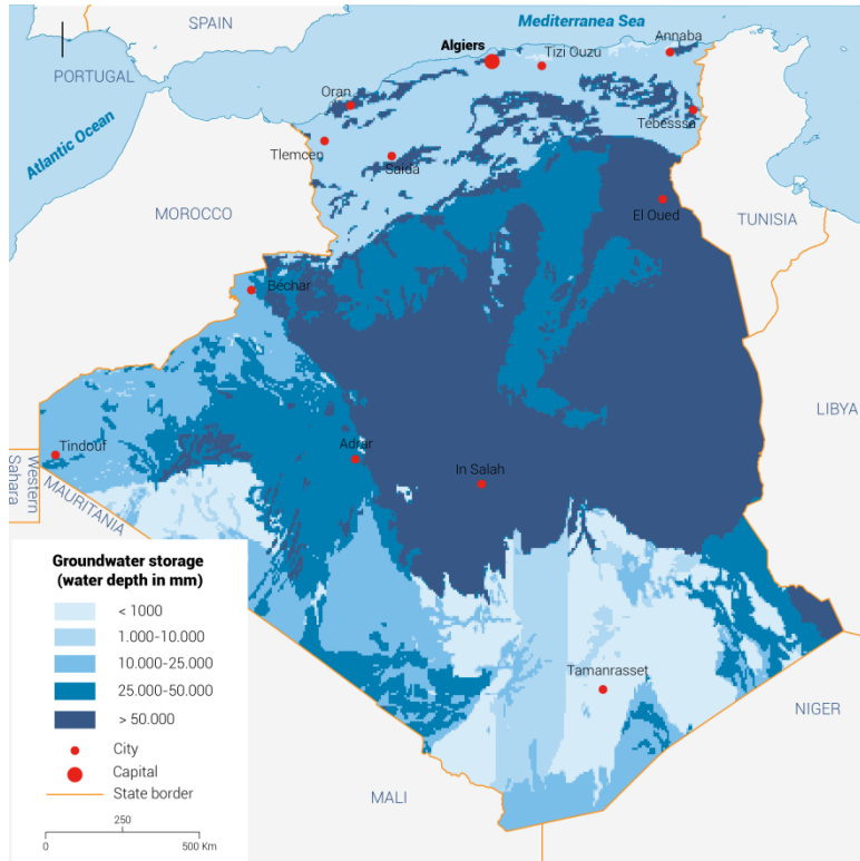
الشكل 3.2: خريطة المياه الجوفية في الجزائر.
