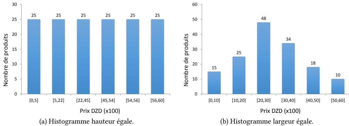
FIGURE 2.15 – Exemples des histogrammes de distribution des valeurs d'attribut Prix de la table Produit .
