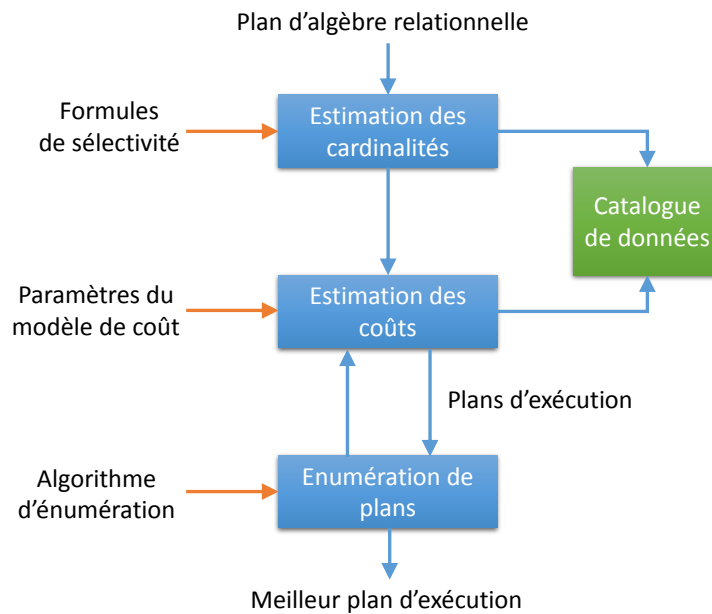
FIGURE 2.14 – Une architecture globale pour l'étape d'optimisation de requêtes.
