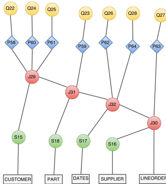
FIGURE 6.2 – Exemple d'un \mathcal{GGR} de 7 requêtes.
