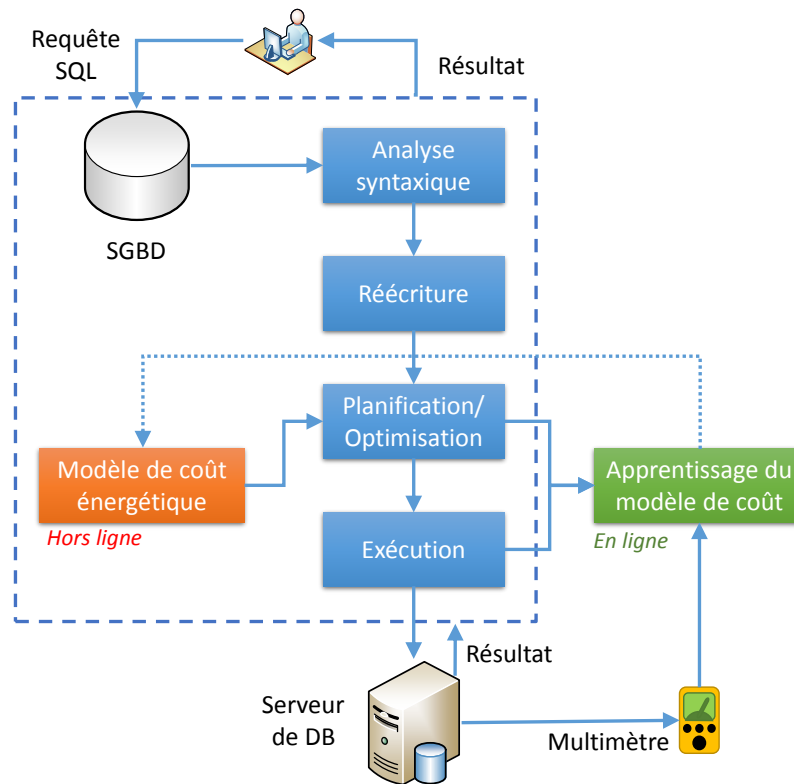
FIGURE 5.3 – La méthodologie de conception
