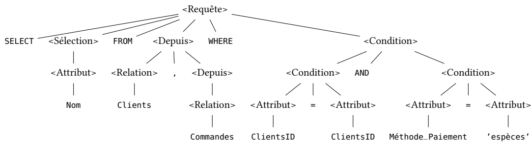
FIGURE 2.11 – Exemple d'un arbre d'analyse.
