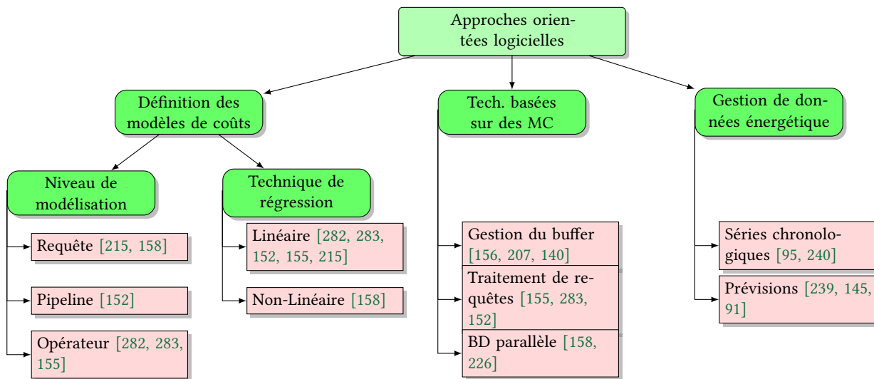
FIGURE 3.5 – Classification des approches d'EE orientées logicielles.
