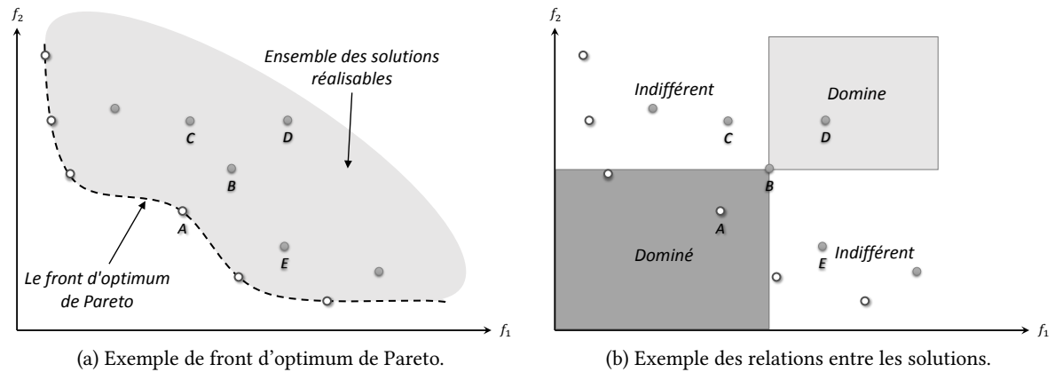
FIGURE 2.18 – Exemples de la notion de dominance de Pareto dans l'espace objectif.
