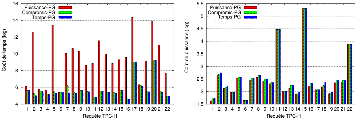
FIGURE 5.13 – Performance et puissance pour les requêtes de TPC-H en utilisant différentes configurations de EnerQuery .
