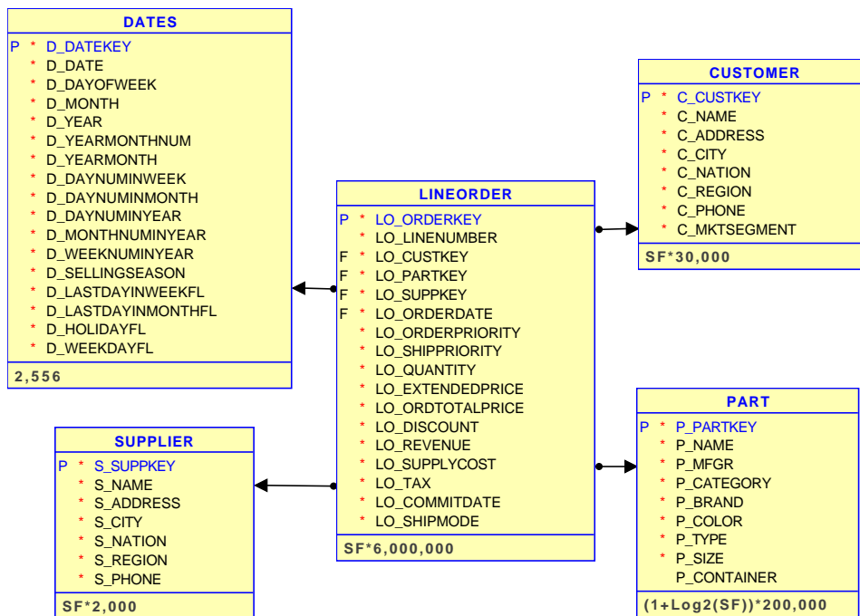
FIGURE 6.6 – Schéma du benchmark SSB.
