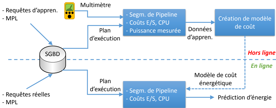
FIGURE 4.6 – Le processus de conception du modèle de coût énergétique.
