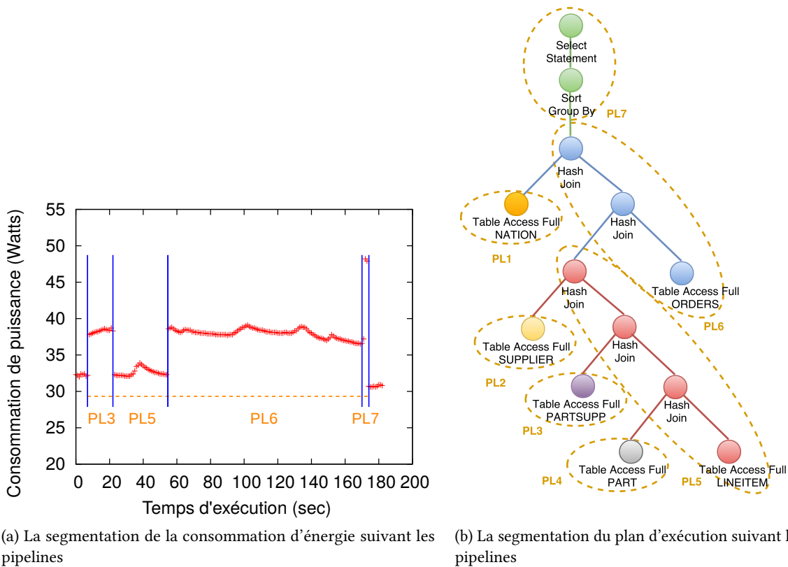
FIGURE 4.4 – La consommation d'énergie et le plan d'exécution de la requête Q_9 issue du benchmark TPC-H avec l'annotation des pipelines correspondante.
