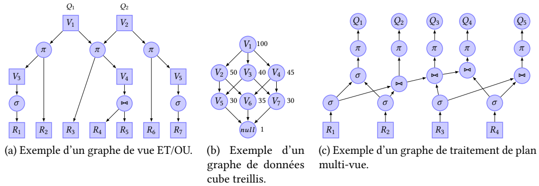
FIGURE 2.8 – Des exemples de structures de données graphe orienté acyclique.
