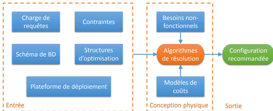
FIGURE 6.1 – Schéma de la conception physique des bases de données.
