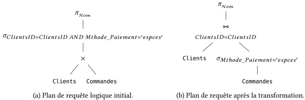
FIGURE 2.13 – Transformation du plan de requête logique pour l'Exemple 5.
