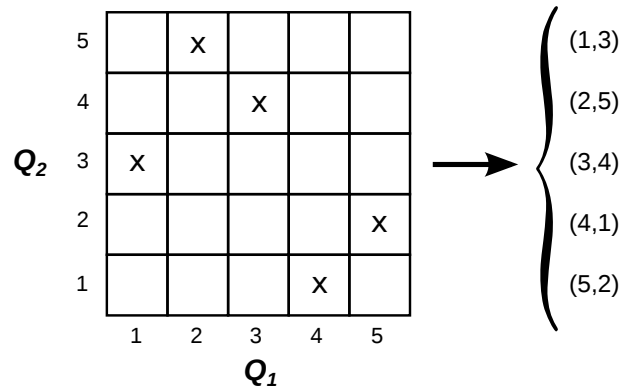
FIGURE 4.18 – Exemple d'échantillonnage par hypercube latin en 2-D.
