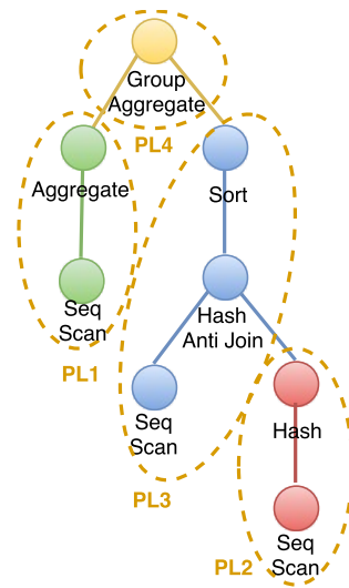
FIGURE 5.2 – Plan d'exécution de la requête Q22 issue du benchmark TPC-H avec l'annotation de pipeline correspondante.
