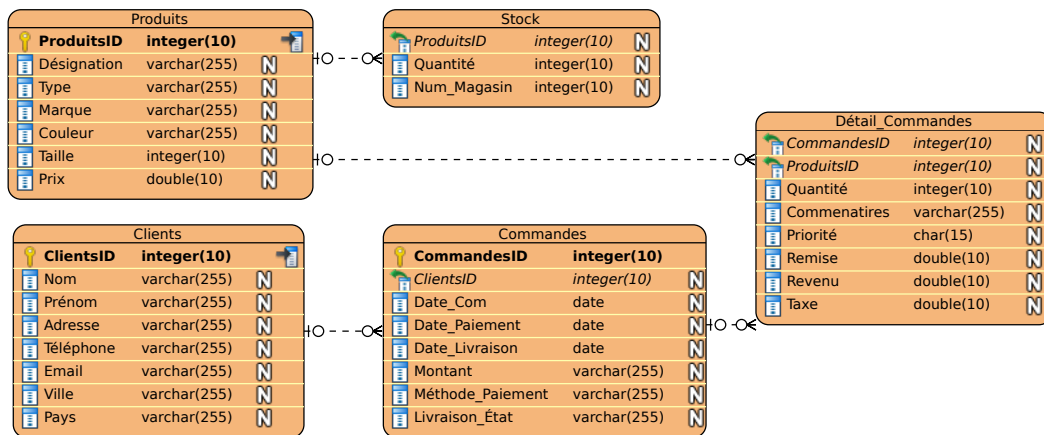
FIGURE 2.6 – Exemple d’un schéma de modélisation physique.
