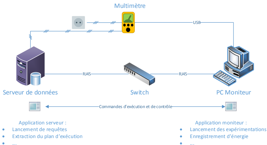
FIGURE 4.13 – Applications de gestion d'expérimentations.
