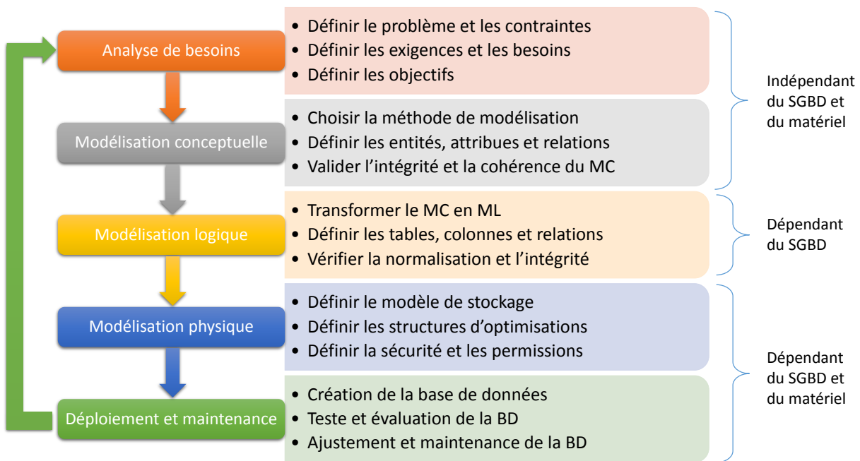
FIGURE 2.2 – Le cycle de vie des bases de données.
