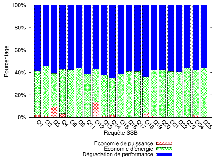
FIGURE 6.13 – Impact des configurations de vues matérialisées sur les performances et la consommation d'énergie des requêtes SSB.
