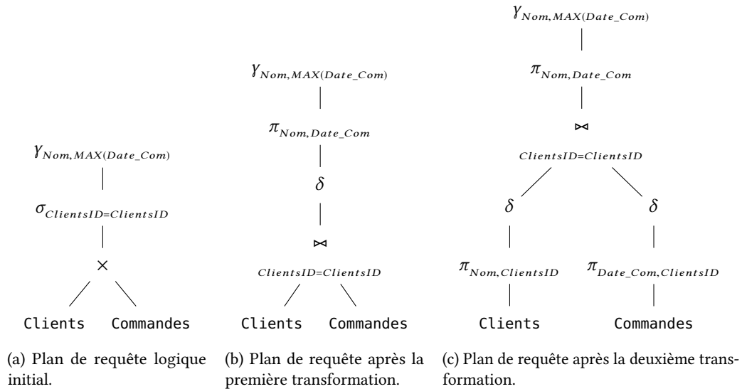
FIGURE 2.12 – Étape de transformation du plan de requête logique pour l'Exemple 6.
