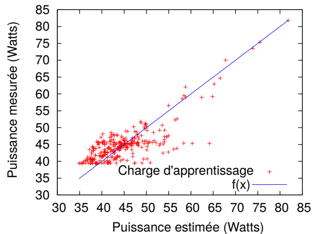
FIGURE 4.17 – La qualité de la régression polynomiale pour la phase d’apprentissage du modèle de coût énergétique en mode concurrent.
