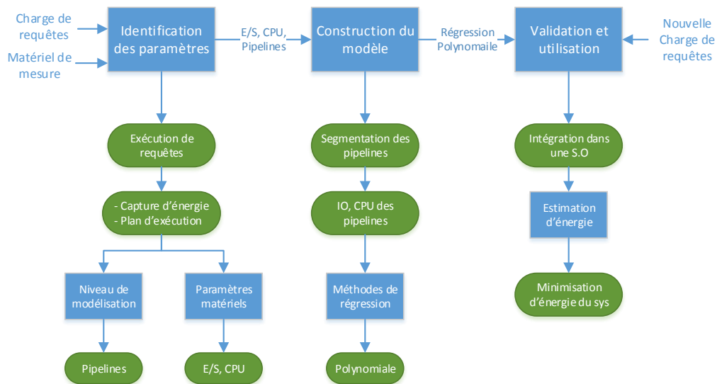
FIGURE 4.12 – Vue d'ensemble sur le modèle de coût énergétique.
