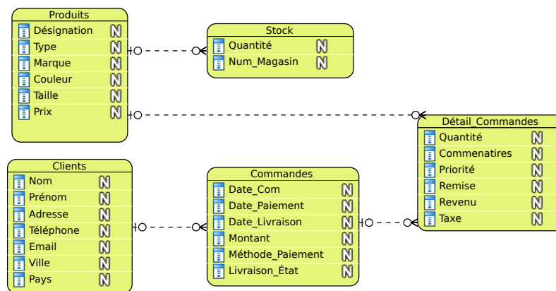
FIGURE 2.4 – Exemple d'un schéma de modélisation conceptuelle.
