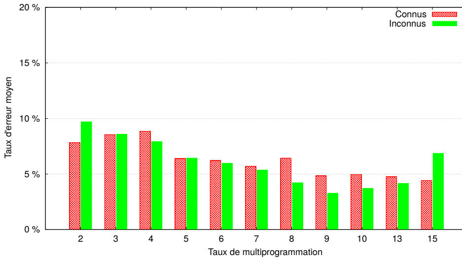
FIGURE 4.19 – Erreurs d'estimation d'énergie dans le benchmark TPC-H pour les modèles de requêtes connus et inconnus.
