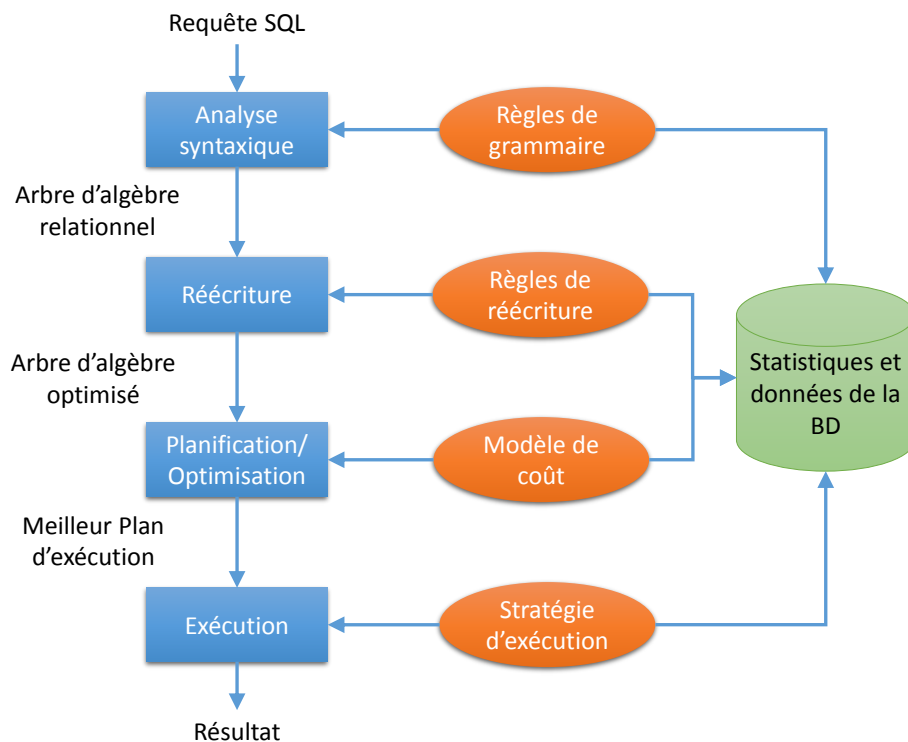
FIGURE 5.1 – Étapes de traitement de requêtes dans PostgreSQL.
