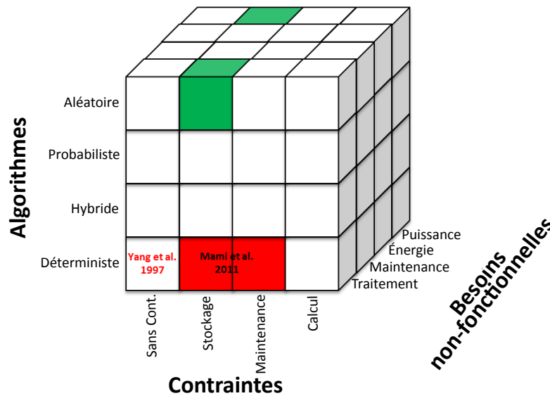
FIGURE 2.7 – Méthodes de résolutions du \mathcal{PSV} .
