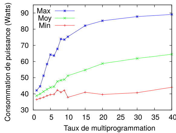
FIGURE 4.5 – Variation de la consommation d’énergie de la charge de requêtes suivant les différents taux de multiprogrammation (MPLs).
