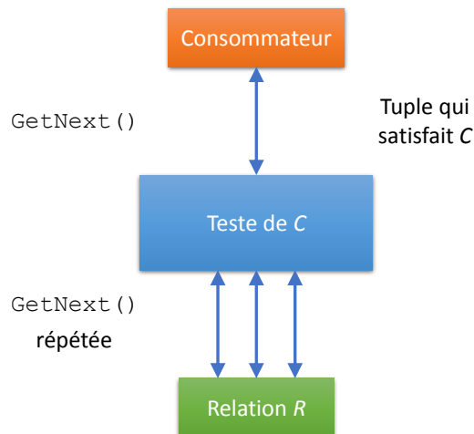
FIGURE 2.17 – Exécution d’une sélection en mode pipeline à l’aide d’itérateurs.
