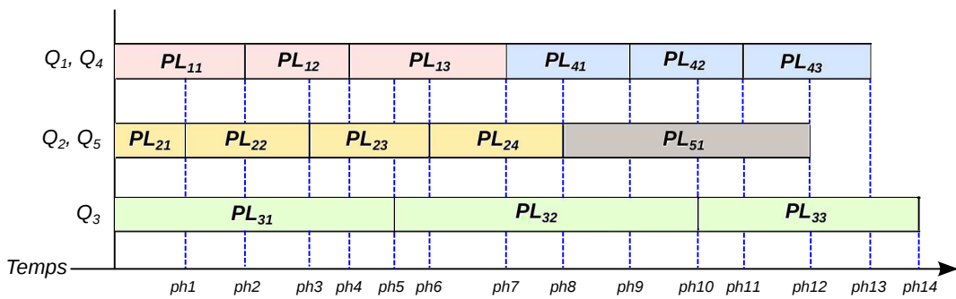
FIGURE 4.8 – Les segmentation des pipelines d'une charge de requêtes concurrentes.
