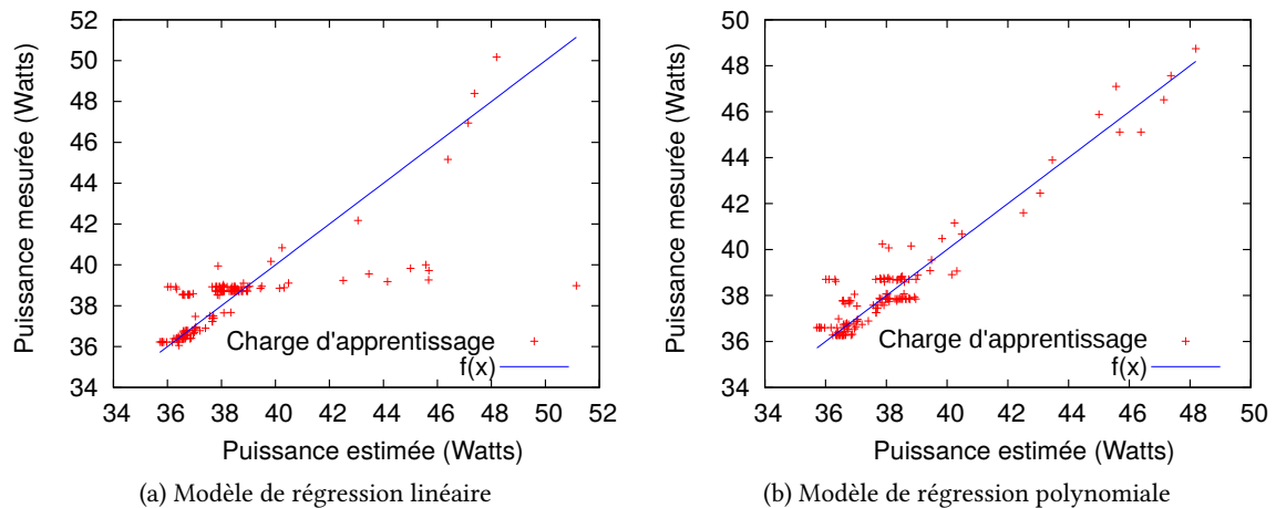
FIGURE 4.15 – La qualité des méthodes de régressions pour la phase d'apprentissage du modèle de coût énergétique.
