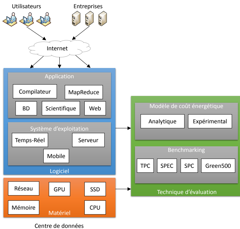
FIGURE 3.2 – La consommation d'énergie dans les systèmes informatiques sur les trois niveaux.
