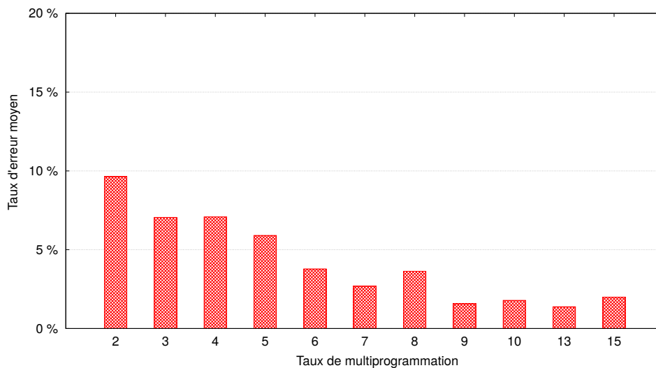
FIGURE 4.21 – Erreurs d’estimation d’énergie dans le benchmark TPC-H pour tous les modèles de requêtes.
