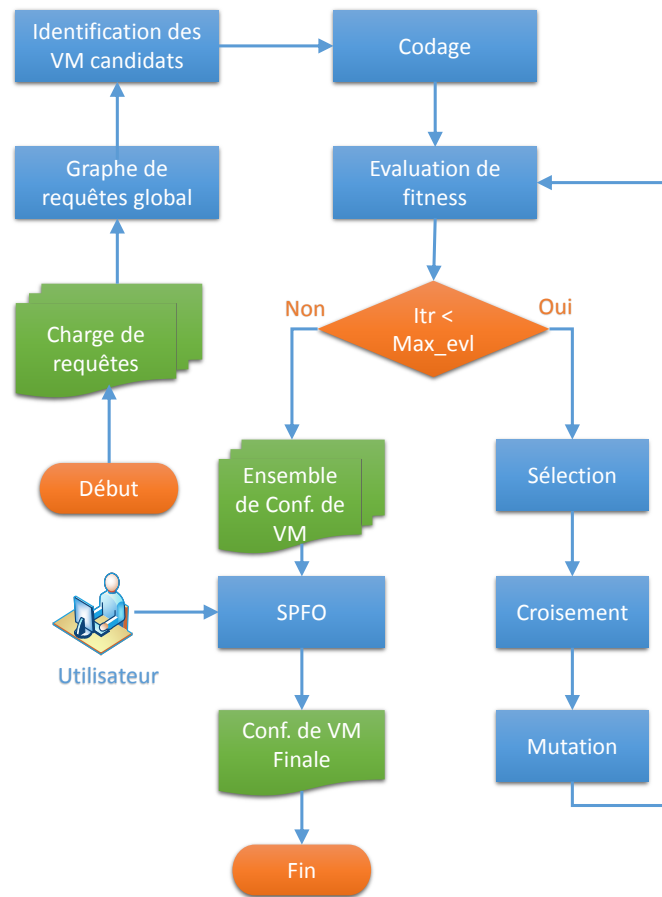
FIGURE 6.5 – Le processus de sélection des vues.
