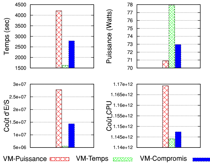
FIGURE 6.9 – Les caractéristiques des vues matérialisées et leurs impacts sur la performance et la consommation d'énergie.
