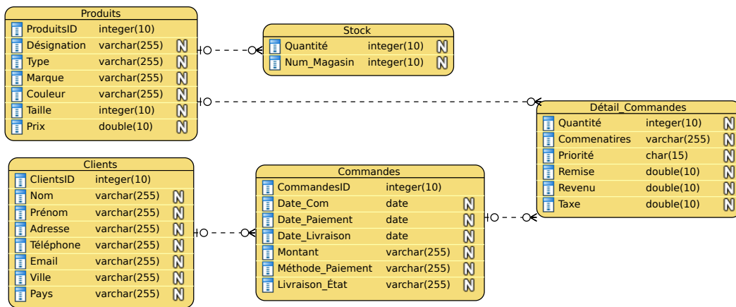
FIGURE 2.5 – Exemple d'un schéma de modélisation logique.
