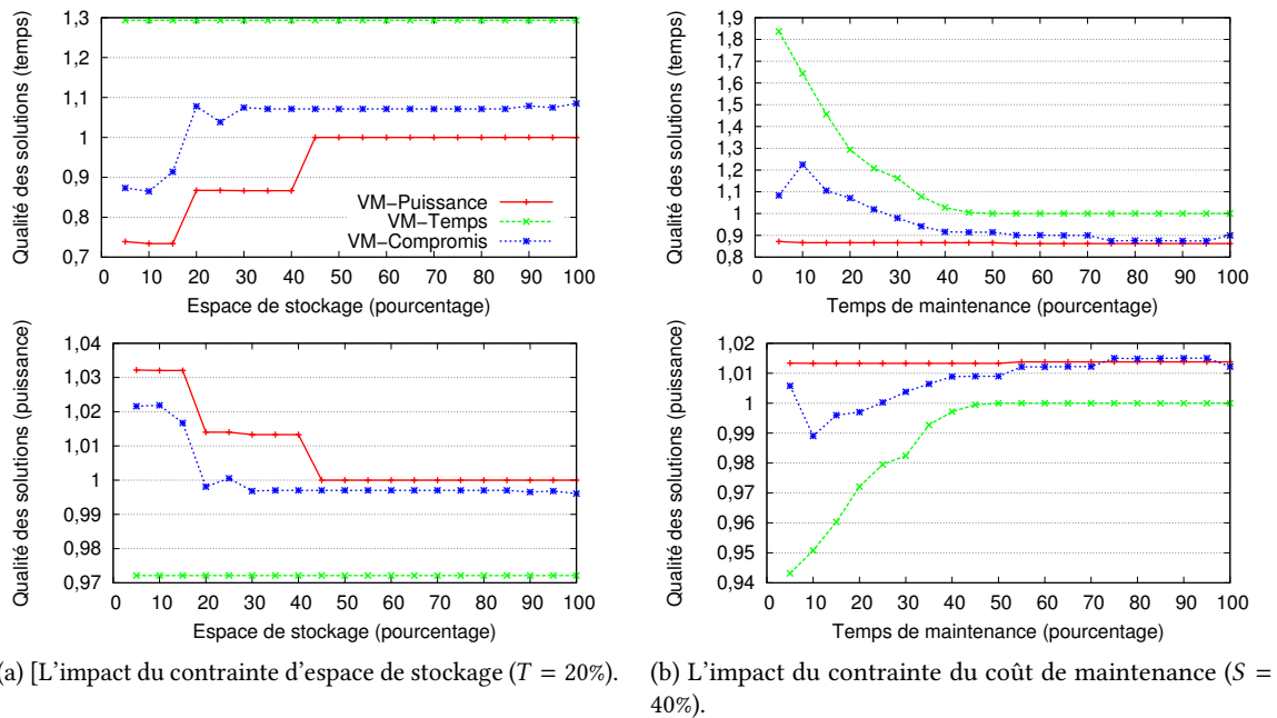
FIGURE 6.11 – Qualité des solutions en terme de performance et de consommation d'énergie avec différentes combinaisons de contraintes.
