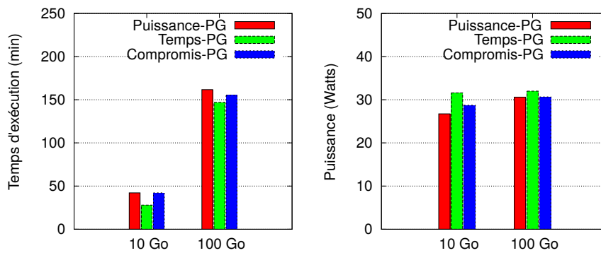
FIGURE 5.14 – Performance et économie d'énergie avec différentes configurations de EnerQuery en utilisant TPC-H.
