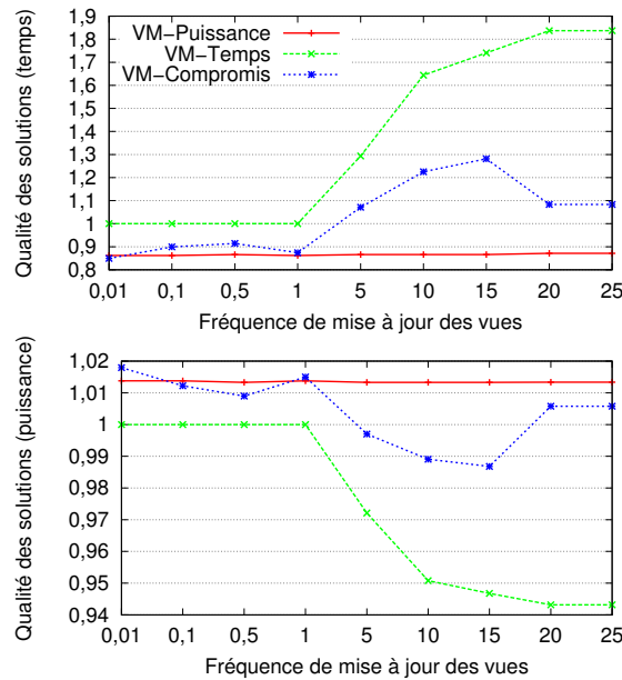
FIGURE 6.12 – Qualité des solutions en terme de performances et de consommation d'énergie avec différentes fréquences de mises à jour ( S = 40\% ).
