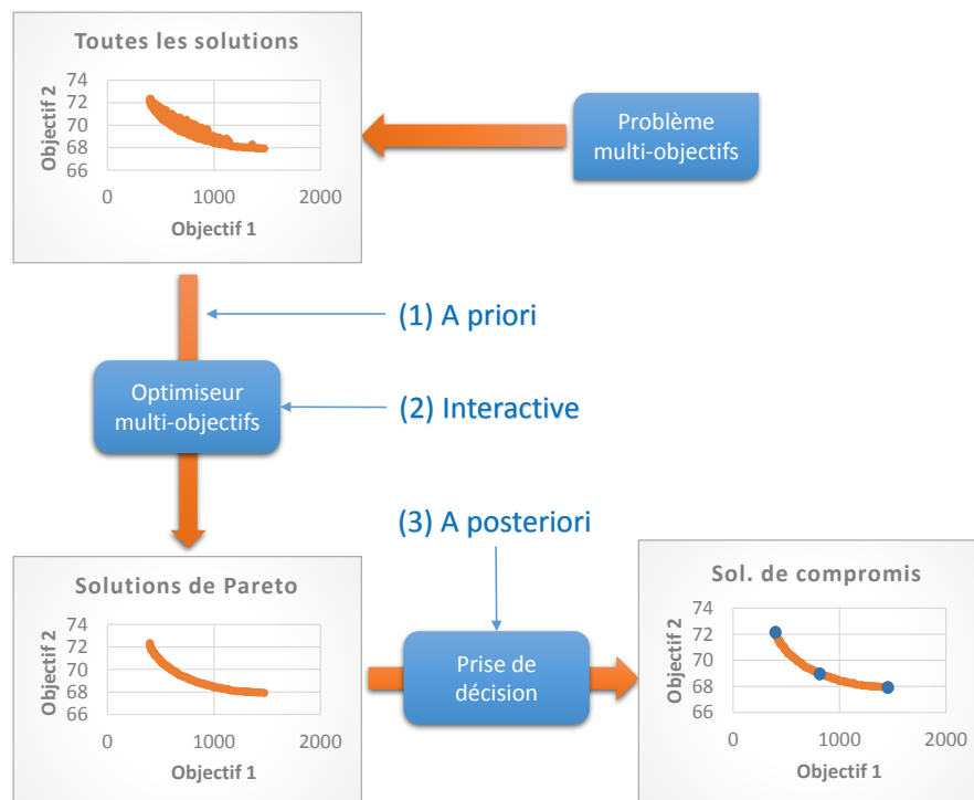
FIGURE 6.4 – Procédé d'application d'optimisation multi-objectifs.
