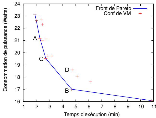
FIGURE 6.3 – Exemple de frontière de Pareto lors de la minimisation de deux objectifs (performance et énergie).
