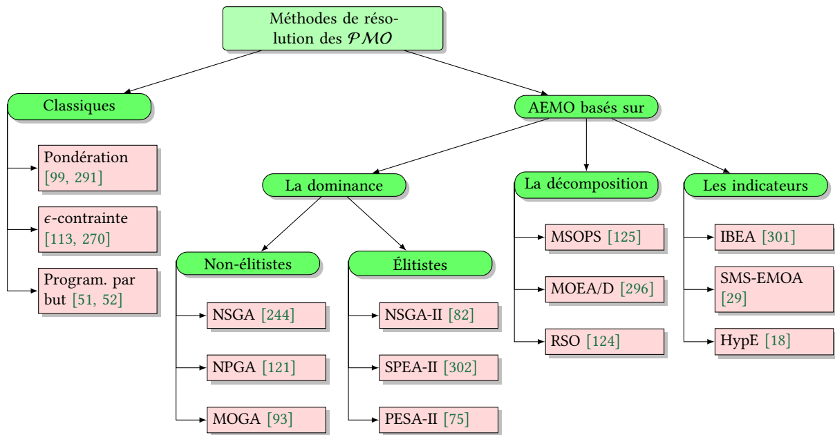
FIGURE 2.22 – Classification des méthodes de résolutions d'un \mathcal{PMO} .
