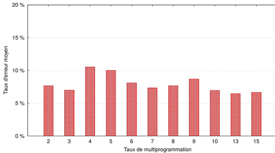
FIGURE 4.20 – Erreurs d’estimation d’énergie dans les requêtes du benchmark TPC-DS en mode concurrent.
