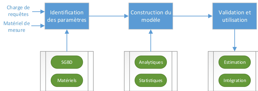
FIGURE 4.2 – Les étapes de développement de notre modèle de coût énergétique.
