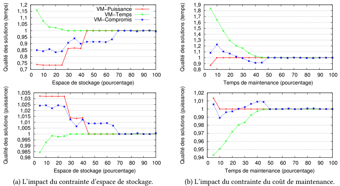
FIGURE 6.10 – Qualité des solutions en terme de performance et de consommation d'énergie avec la contrainte des ressources.
