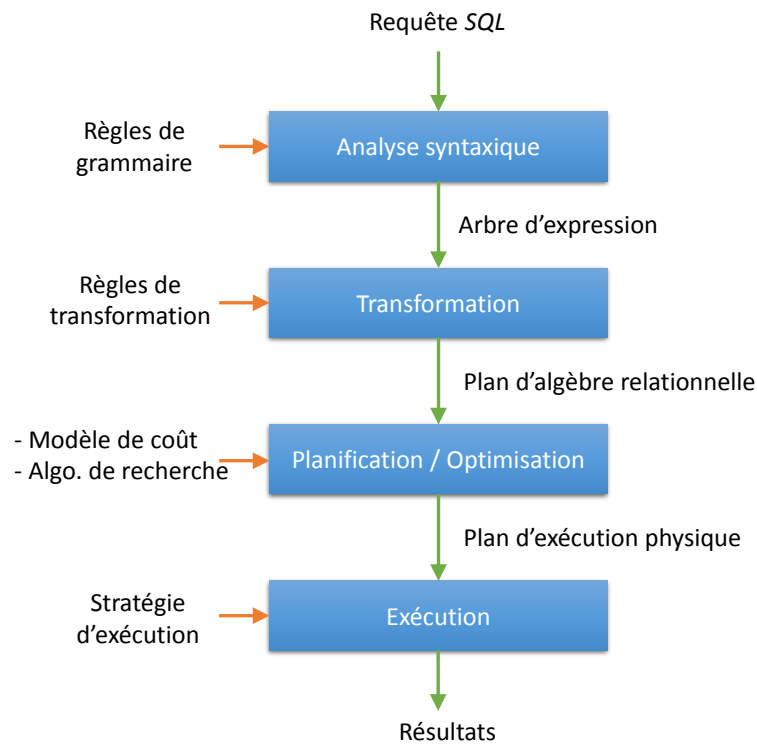
FIGURE 2.10 – Architecture globale pour le traitement de requêtes dans un SGBD.
