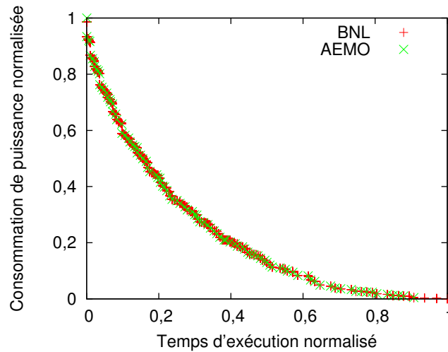
FIGURE 6.8 – Comparaison entre les solutions d'algorithme évolutionnaire et exhaustive.
