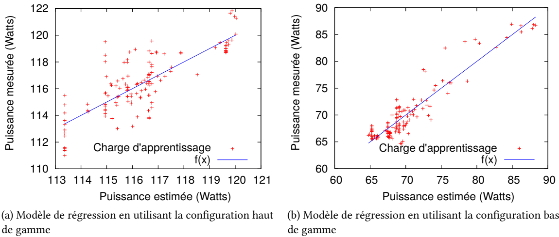
FIGURE 5.12 – La qualité du modèle de coût énergétique avec différent type de machine.
