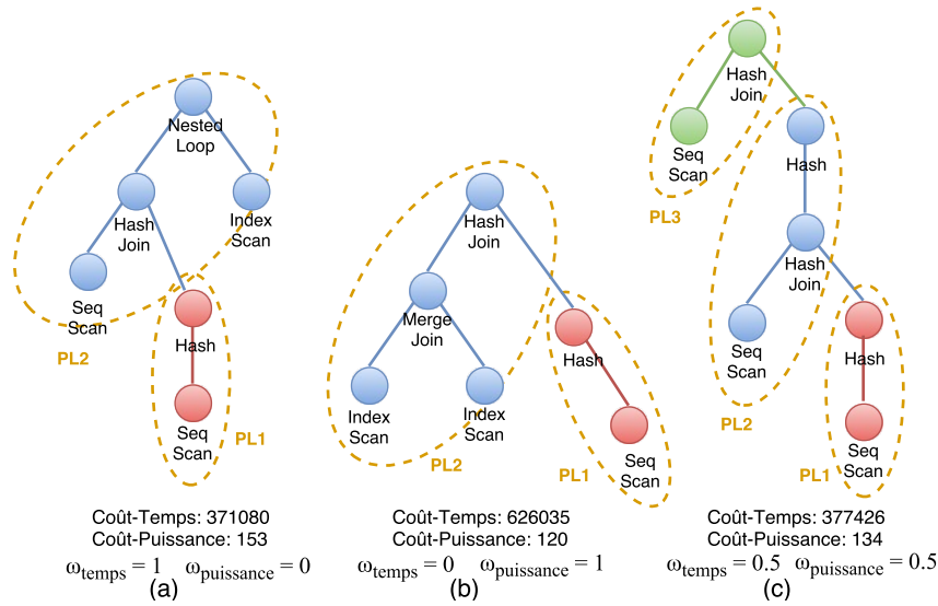
FIGURE 5.4 – Le plan optimal pour la requête Q_3 de TPC-H lors du changement des préférences d'utilisateur.
