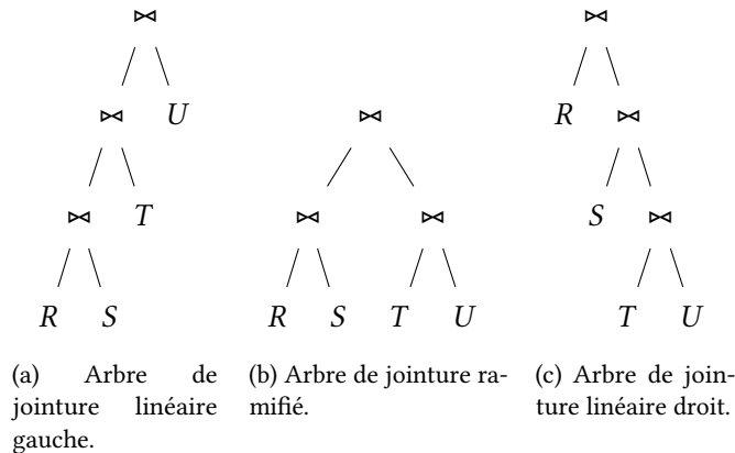
FIGURE 2.16 – Exemple des méthodes pour la jointure de quatre relations.
