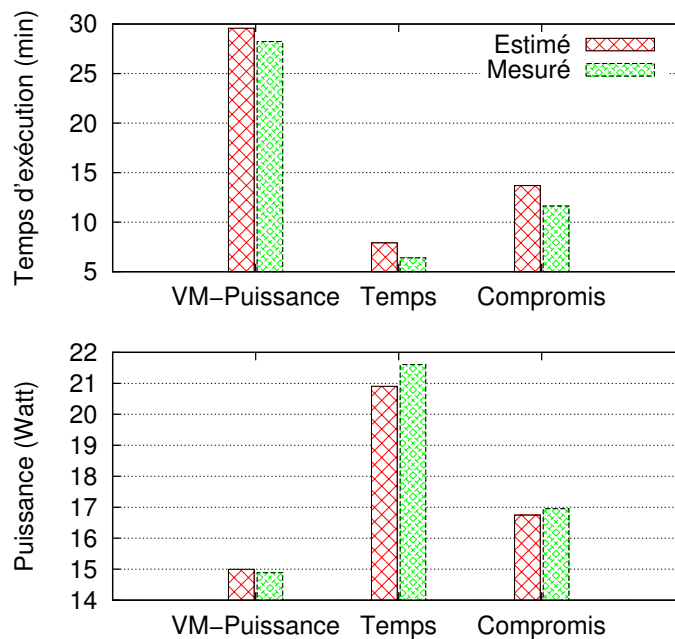
FIGURE 6.7 – Les erreurs d'estimation des performances et de la consommation d'énergie de la charge de requêtes.
