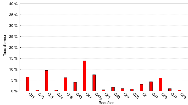
FIGURE 4.16 – Erreurs d'estimation d'énergie dans les requêtes du benchmark TPC-DS.
