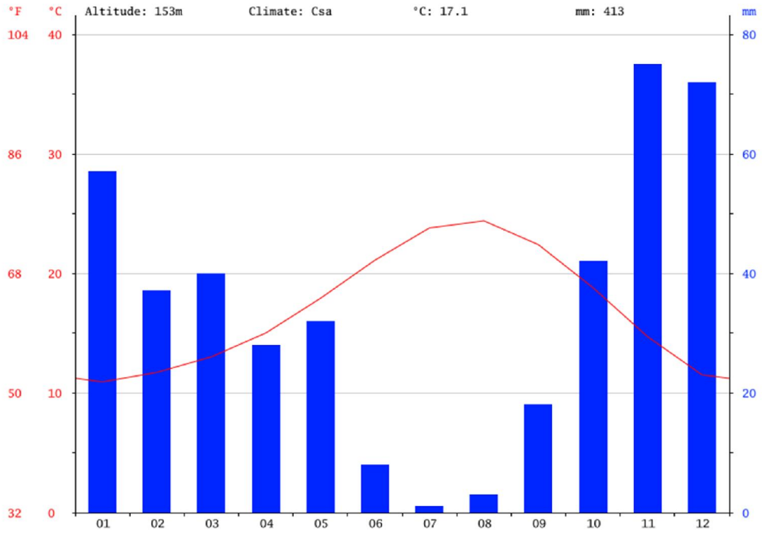
Figure 27 : Diagramme climatique Sidi Ali (CLIMATE-DATA.ORG 2016).
