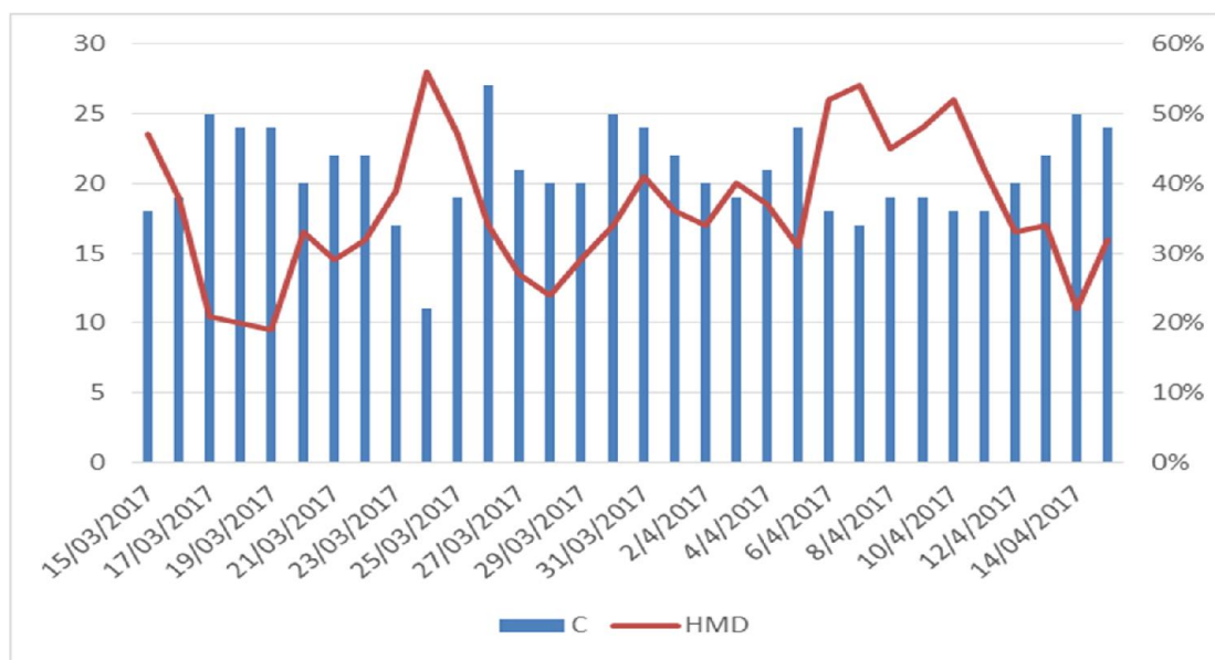
Figure 04 : Diagramme climatique Sidi Ali (CLIMATE-ORG 2017).
