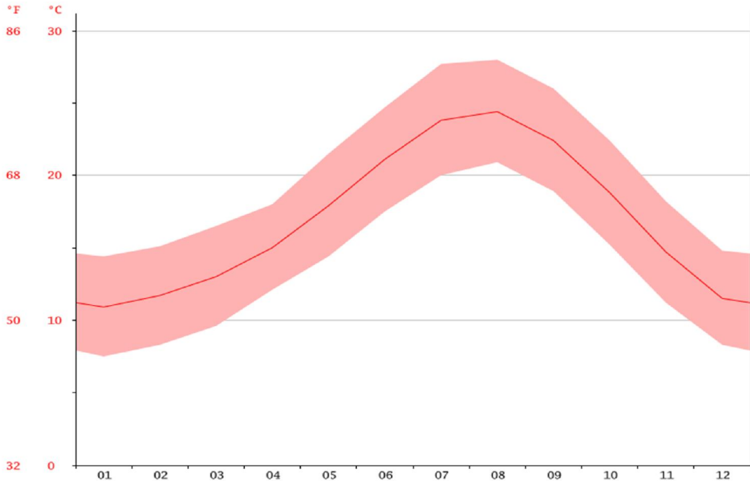
Figure 28 : Courbe de température à Sidi Ali (CLIMATE-DATA.ORG 2016).
