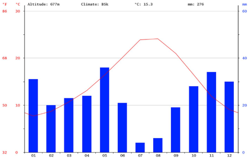
Figure 24 : Diagramme climatique Ain Oussera (CLIMATE-DATA.ORG 2016).
