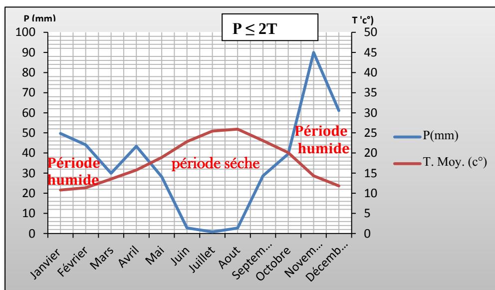
Figure 22. Diagrammes ombrothermique de Bagnoulset Gaussen
