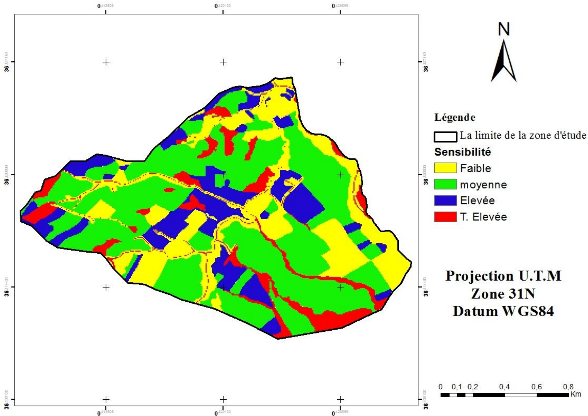
Figure 28. Carte de sensibilité selon le couvert végétal.
