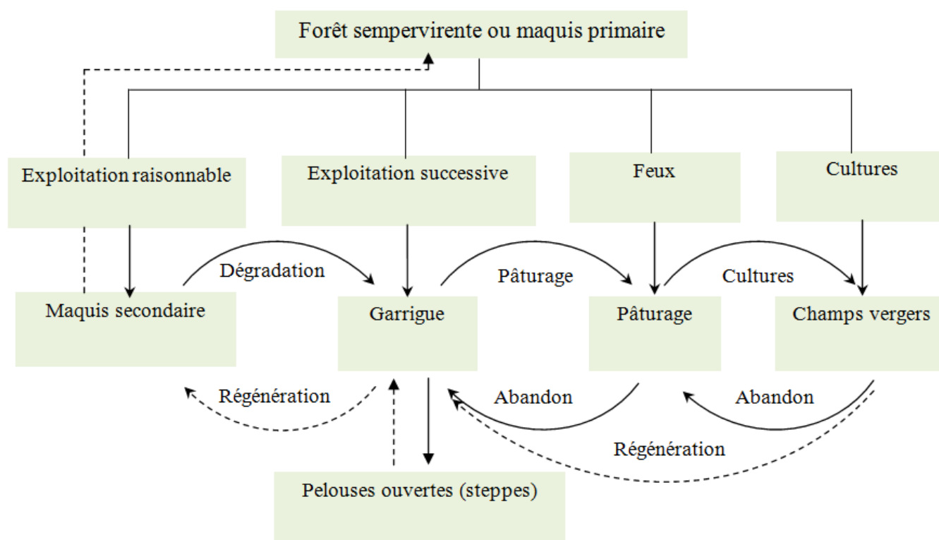
Figure 4. Etapes de la dynamique des peuplements végétaux soumis à l'action de l'homme en région méditerranéenne (d'après Polunin et Huxley, 1965 in Ammar Khoudja, 1986).
