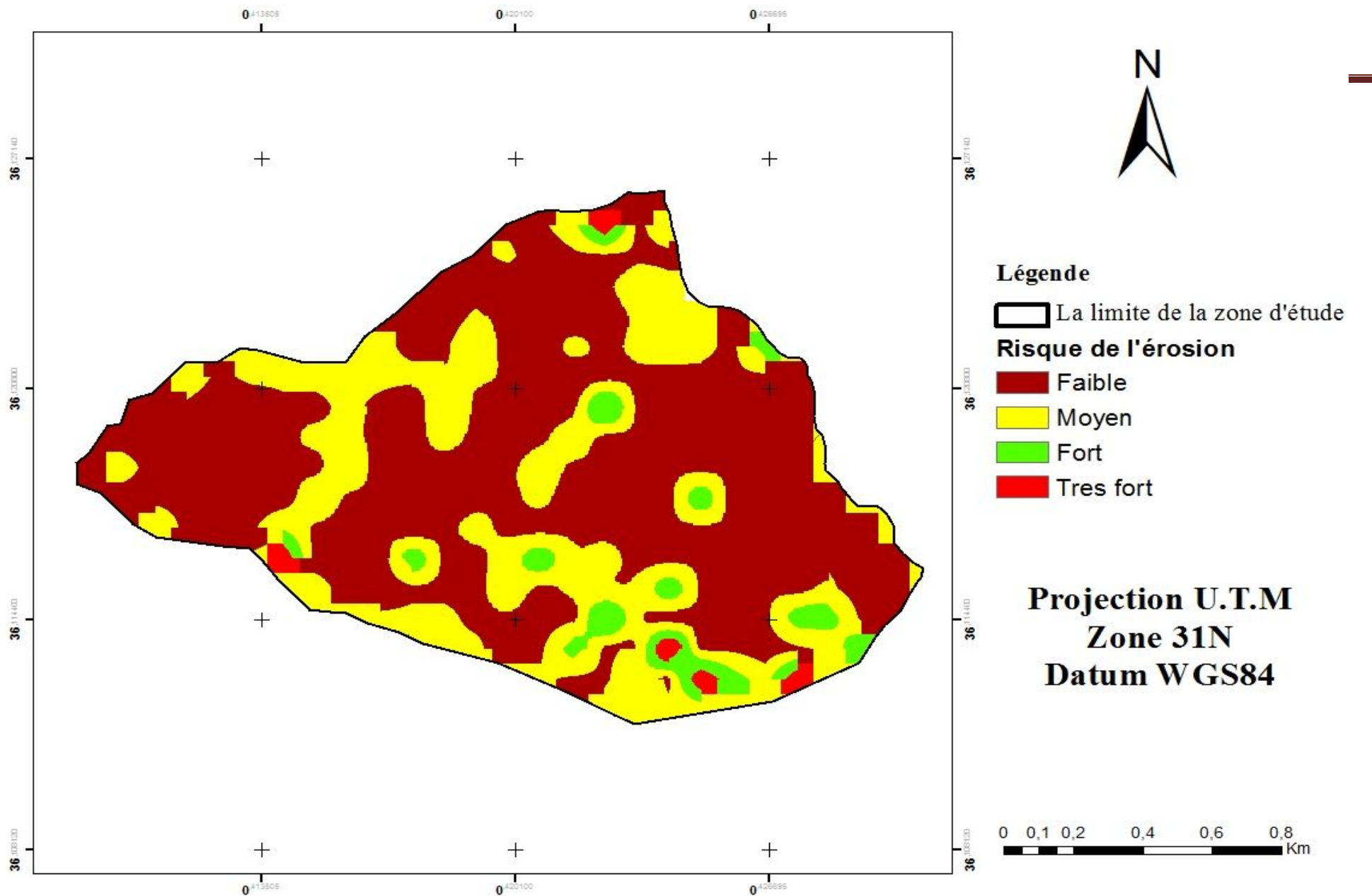
Figure.31 Carte du risque d'érosion.
