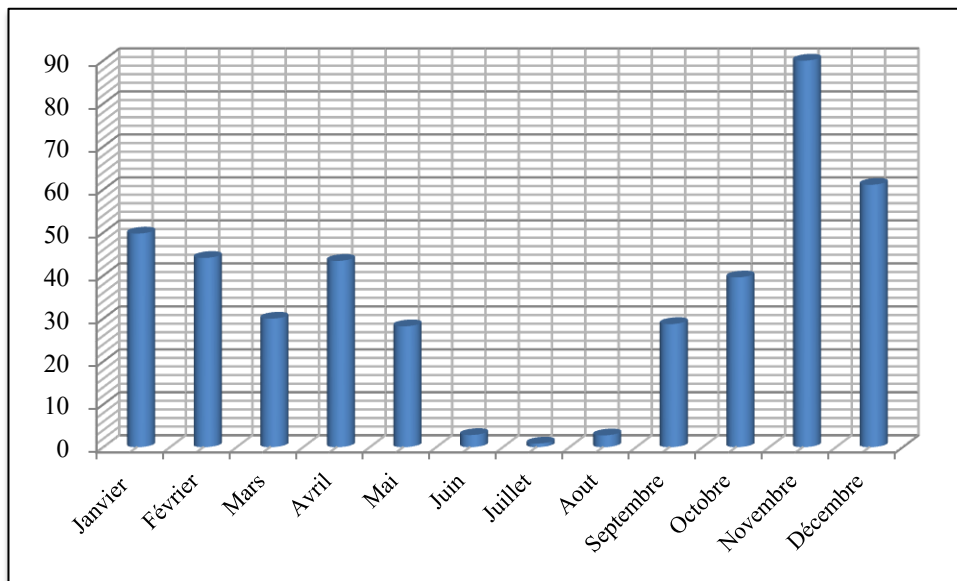
Figure 16. Histogramme des précipitations mensuelles (mm).
