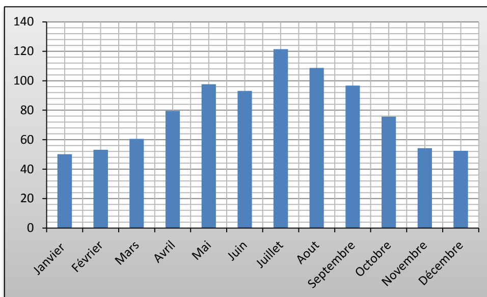
Figure 19. Histogramme de l'évaporation moyenne mensuelle.
