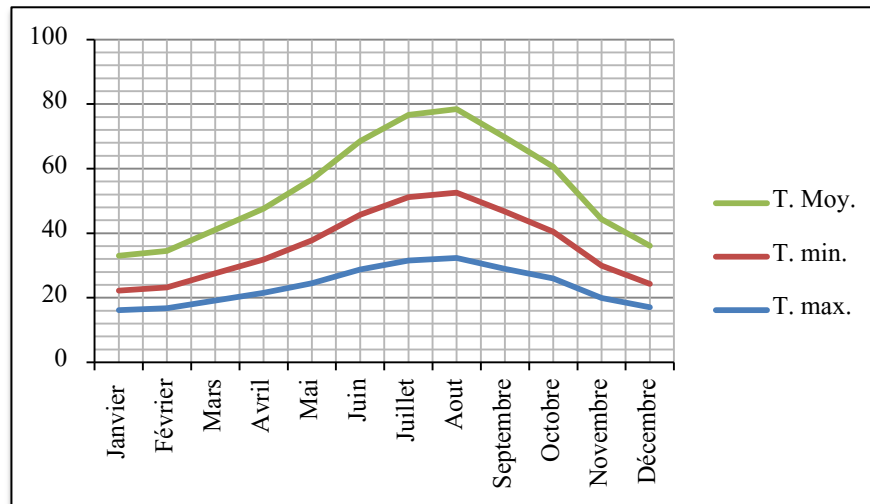
Figure 18. Variations mensuelles des températures moyennes, maximales et minimales.
