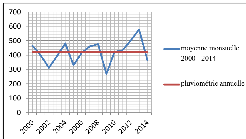
Figure 17. Répartition annuelle de la pluviométrie.
