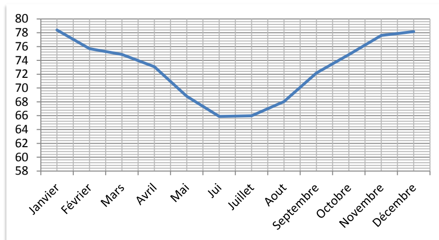
Figure 21. Courbe de la valeur moyenne de l'humidité relative
