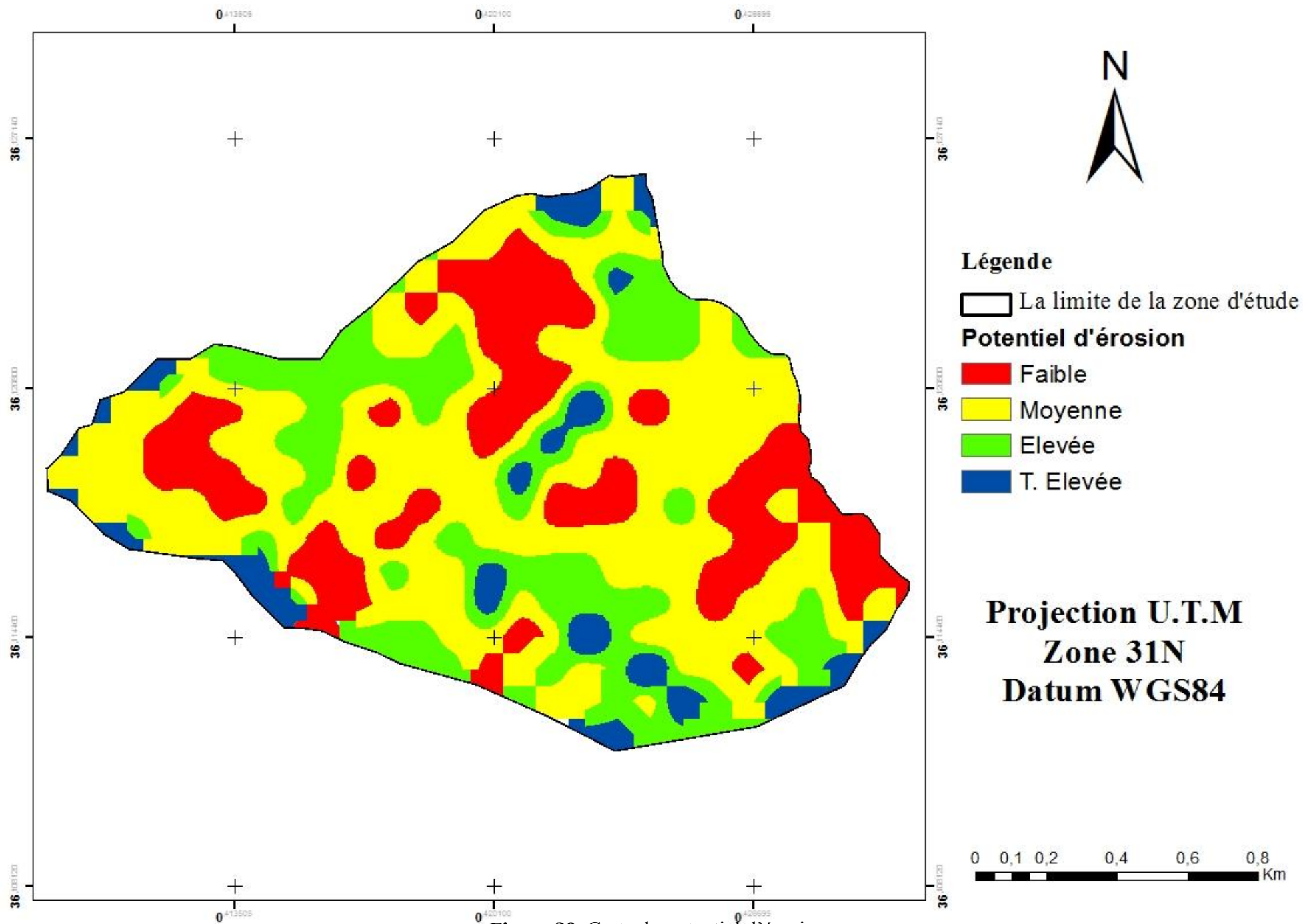
Figure 30. Carte du potentiel d'érosion.
