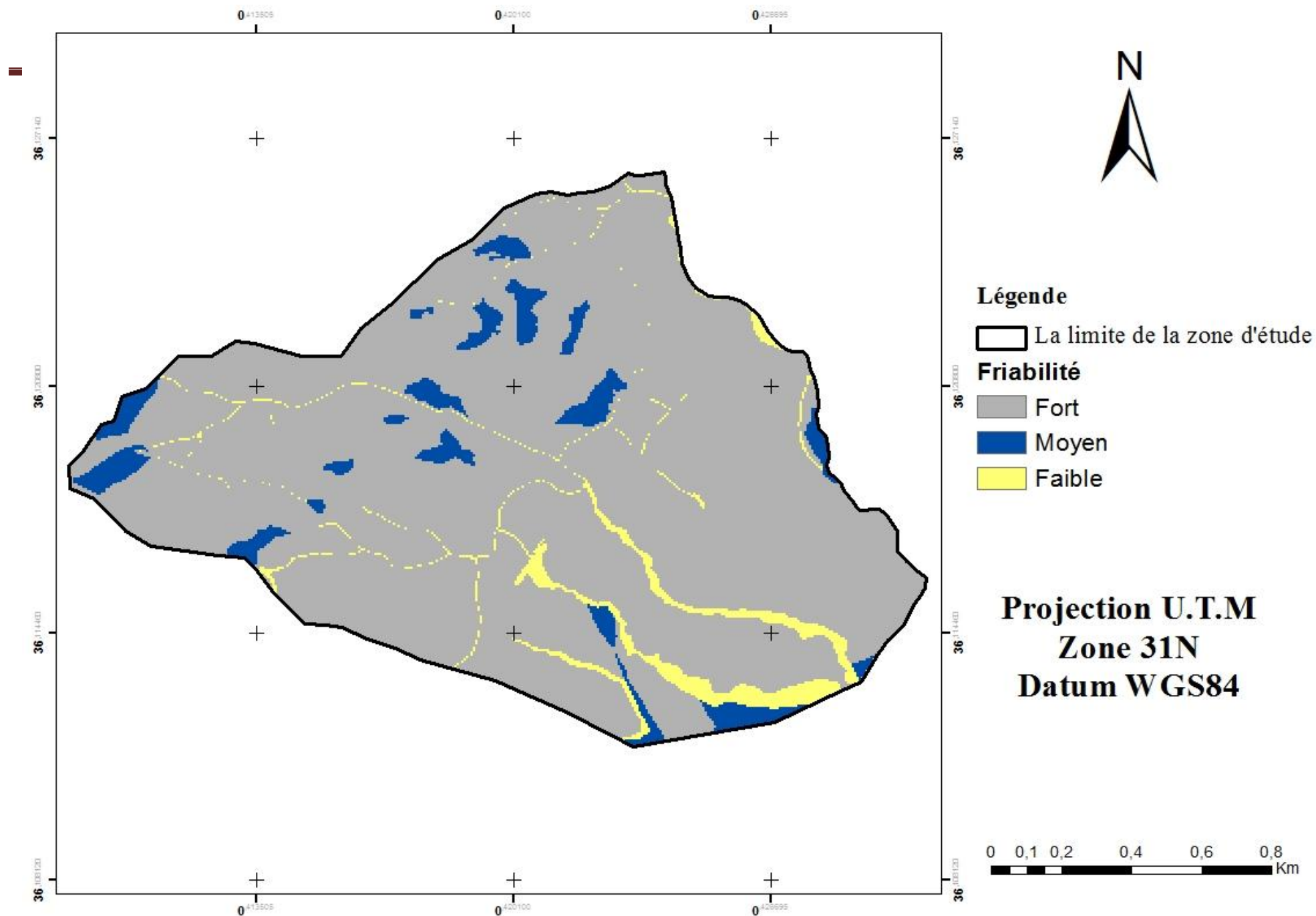
Figure 29. Carte de sensibilité selon la friabilité.
