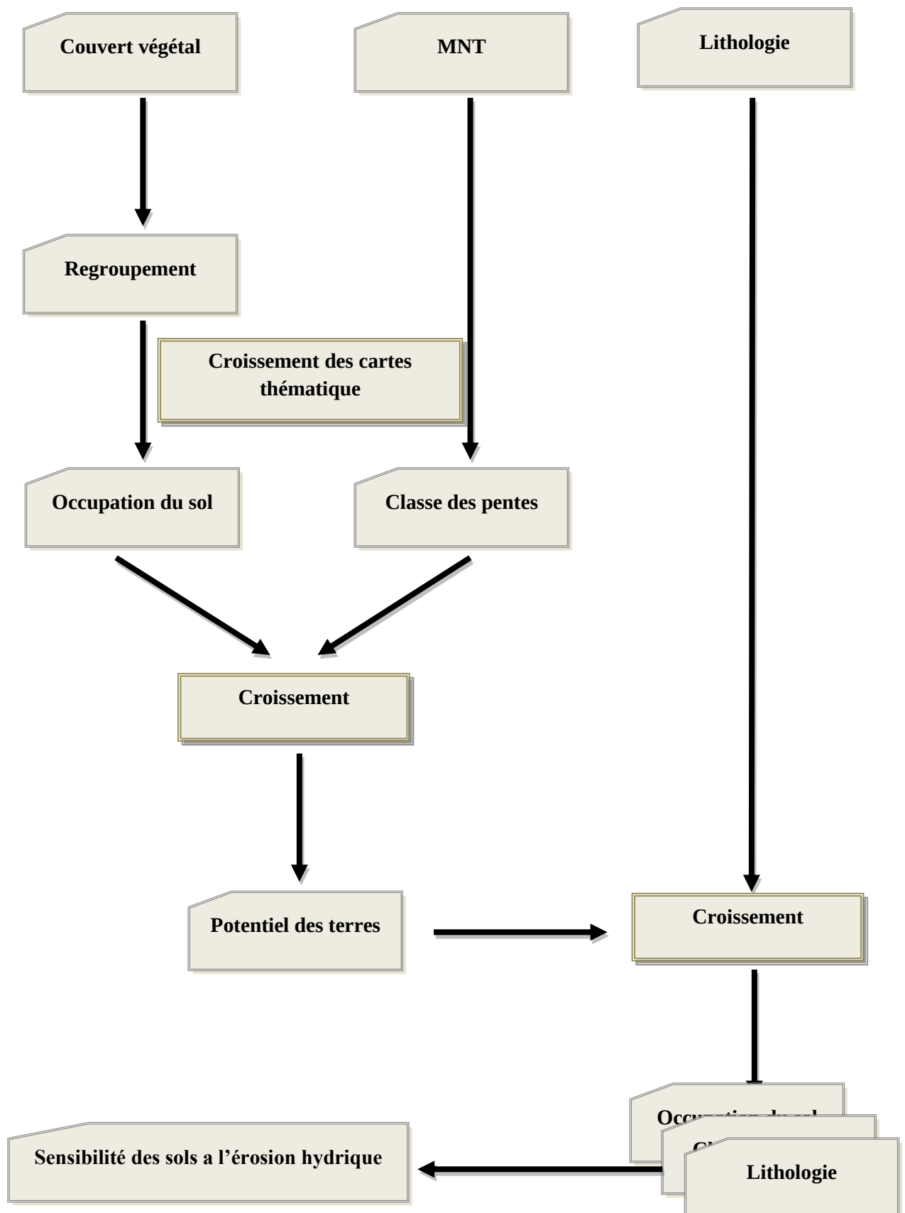
Figure 26. Elaboration des cartes thématiques
