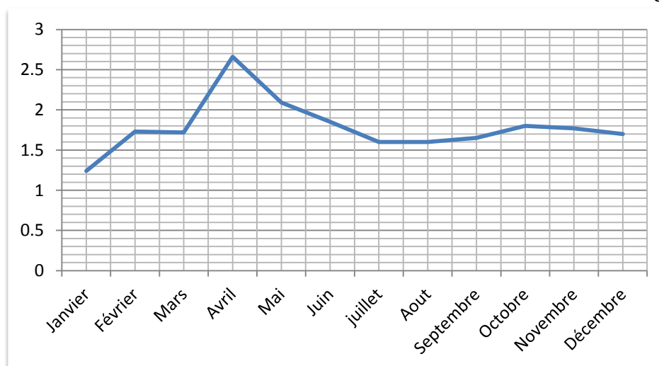
Figure 20. Courbe de la vitesse moyenne mensuelle du vent.
