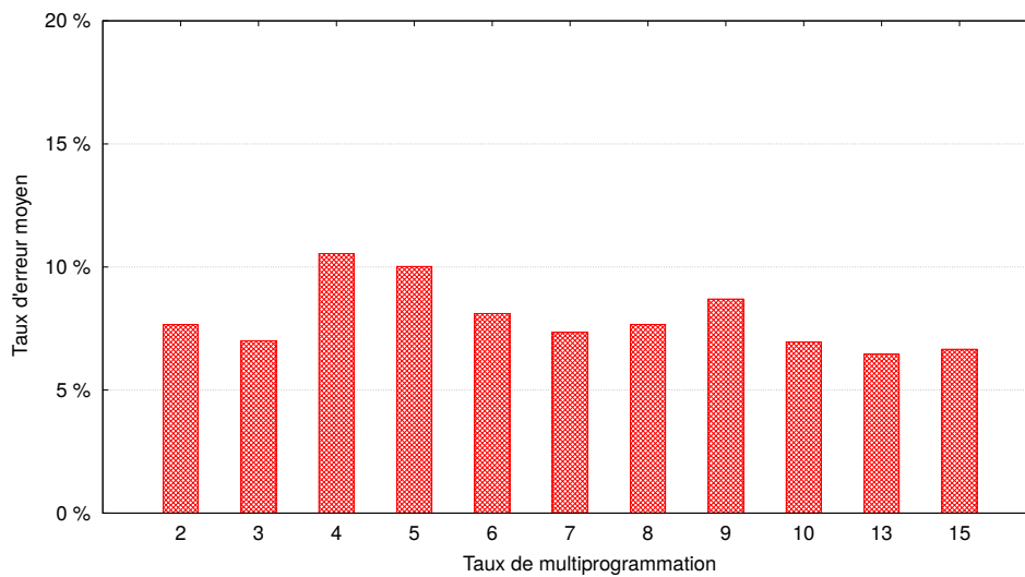
FIGURE 4.20 – Erreurs d’estimation d’énergie dans les requêtes du benchmark TPC-DS en mode concurrent.
