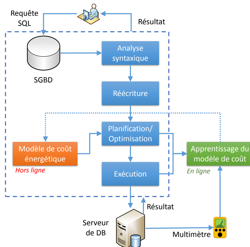
FIGURE 5.3 – La méthodologie de conception
