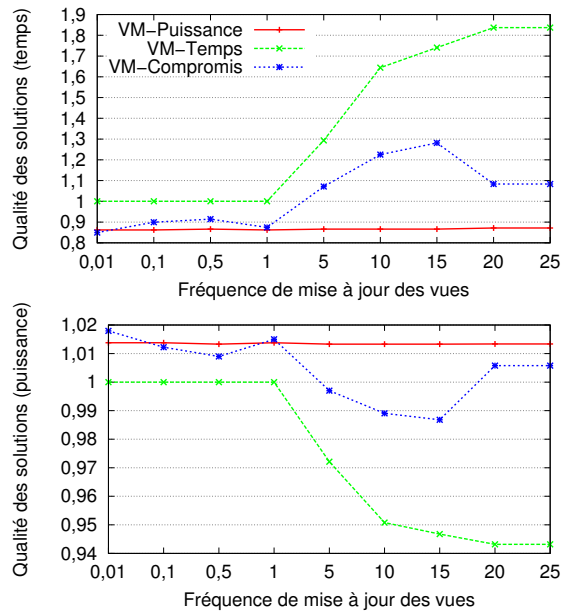
FIGURE 6.12 – Qualité des solutions en terme de performances et de consommation d'énergie avec différentes fréquences de mise à jour ( S = 40\% ).
