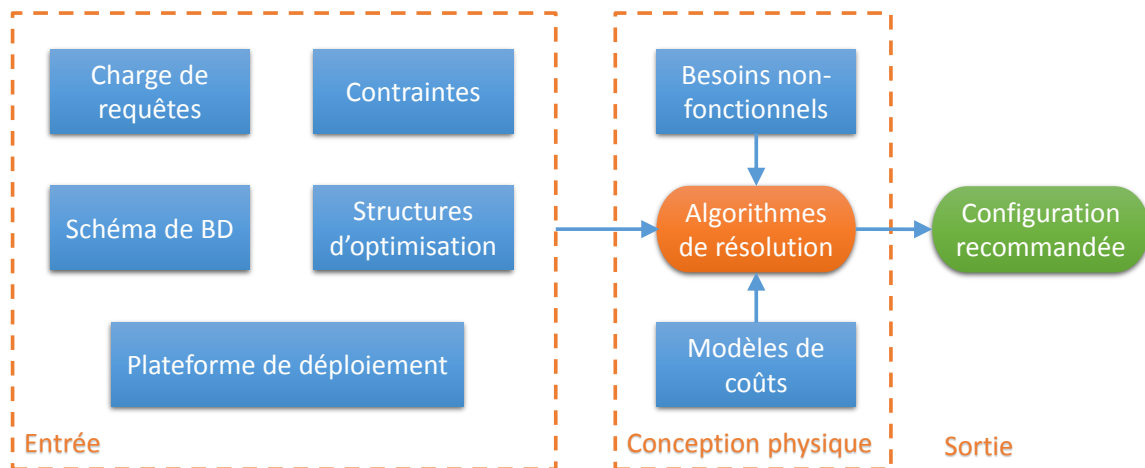
FIGURE 6.1 – Formulation de la conception physique des bases de données.
