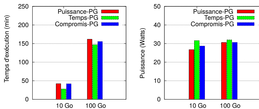
FIGURE 5.14 – Performance et économie d'énergie avec des configurations différentes de EnerQuery en utilisant TPC-H.
