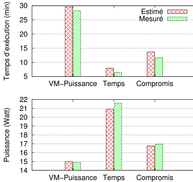
FIGURE 6.7 – Les erreurs d'estimation du performance et consommation d'énergie de la charge de requêtes.
