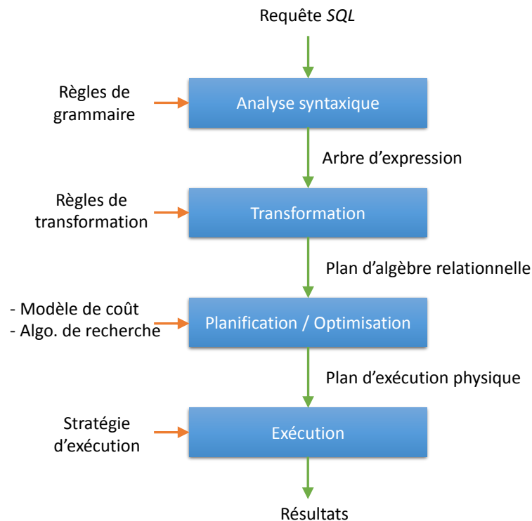
FIGURE 2.10 – Une architecture globale pour le traitement de requêtes dans un SGBD.
