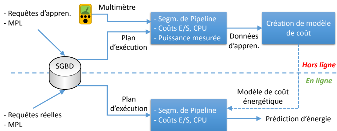
FIGURE 4.6 – Le processus de conception de modèle coût énergétique.
