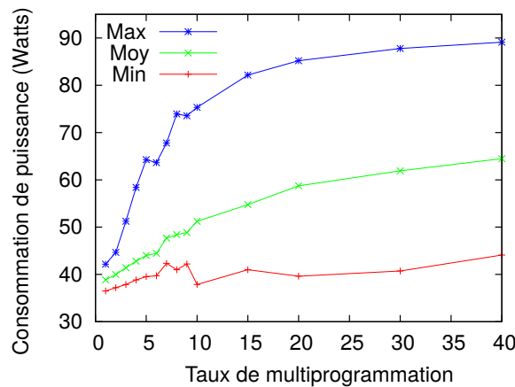
FIGURE 4.5 – Variation de la consommation d'énergie de la charge de travail suivant les différents taux de multiprogrammation (MPLs).
