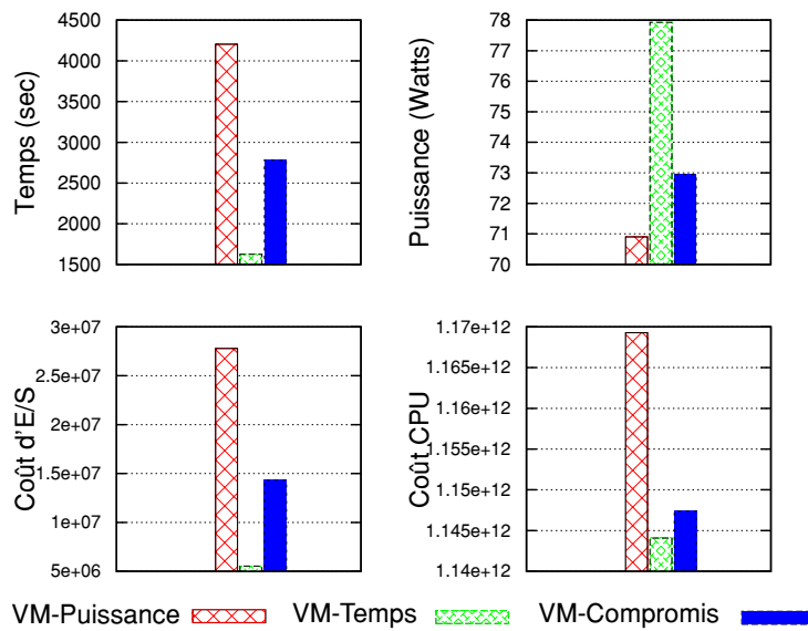
FIGURE 6.9 – Les caractéristiques des vues matérialisées et leur impact sur la performance et la consommation d'énergie.
