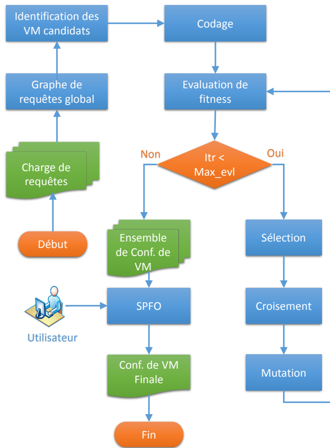
FIGURE 6.5 – Le processus de la méthodologie de sélection de vues.
