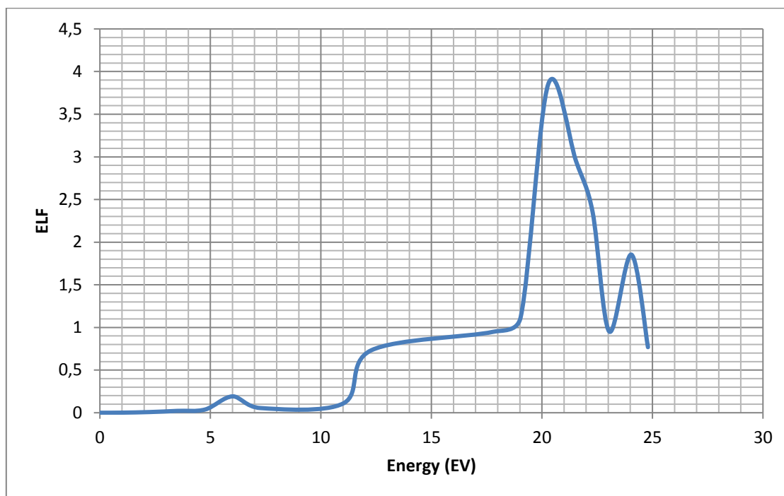
Figure 3.9 : Spectre ELF aux faibles pertes entre 0 et 25 eV et pic de plasmon.
