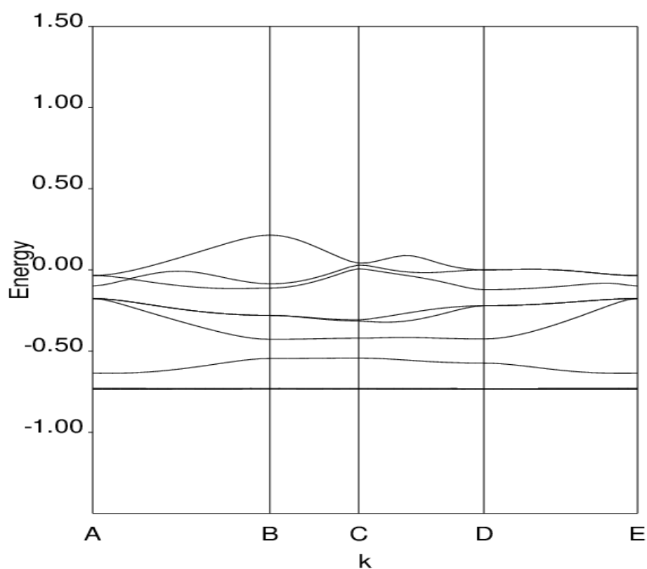
Figure 3.5 : Structure de bandes de GaAs (phase zinc blende)
