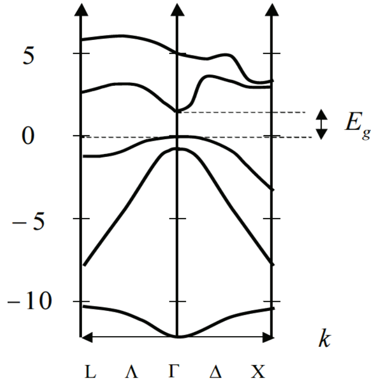
Figure 3.4: structure de bandes suivant les directions principales du GaAs [23,24] La largeur de bande interdite à 300°K est de 1,42 eV.
