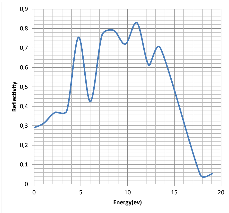
Figure 3.8: Spectre de réflectivité en fonction de l'énergie
