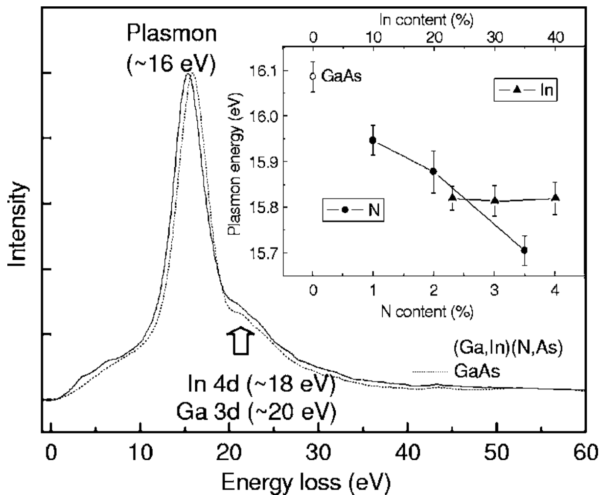
Figure 3.10 : Spectre EELS expérimental aux faibles pertes de GaAs entre 0 et 40 eV et pic de plasmon
