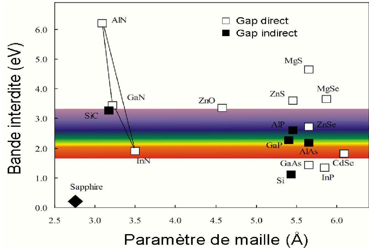
Figure 3.3 : Énergie de la bande interdite en fonction du paramètre de maille à 300°K de différents semi-conducteurs
