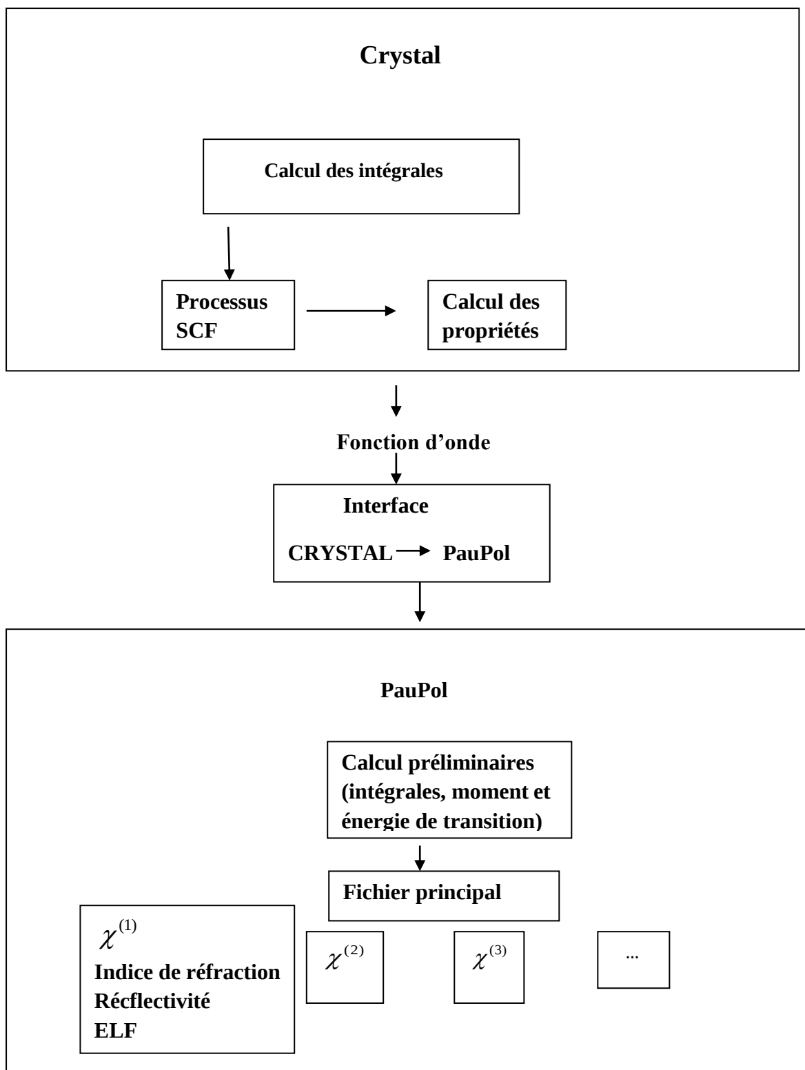
Figure 3.6– Synoptique de la chaîne de calcul CRYSTAL
