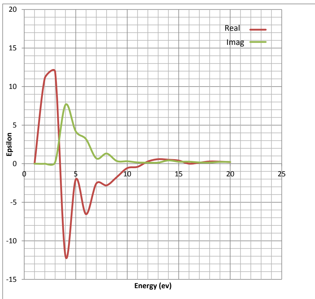
Figure 3.7: Variation de la partie réelle et imaginaire de la fonction diélectrique \epsilon en fonction de l'énergie.
