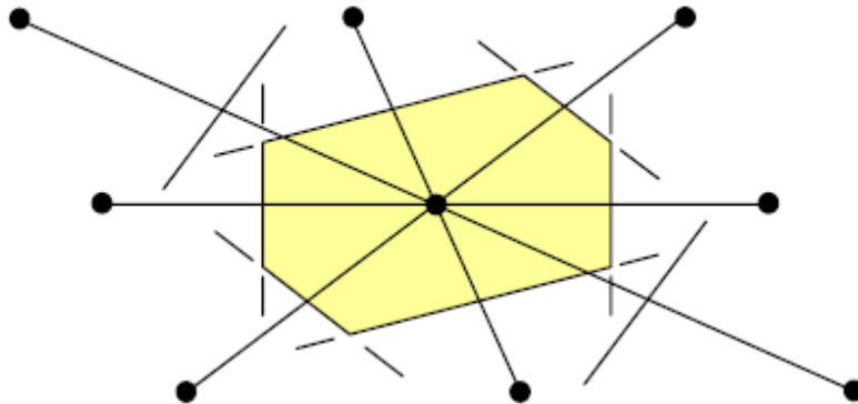
Figure 1.1 : construction de la maille de Wigner-Seitz : a) On trace toutes les directions d'un nœud avec tous ses voisins b) On en déduit les plans médiateurs correspondant à ces directions c) Le plus petit volume enfermé par ces plans est la maille de WIGNER-SEITZ
