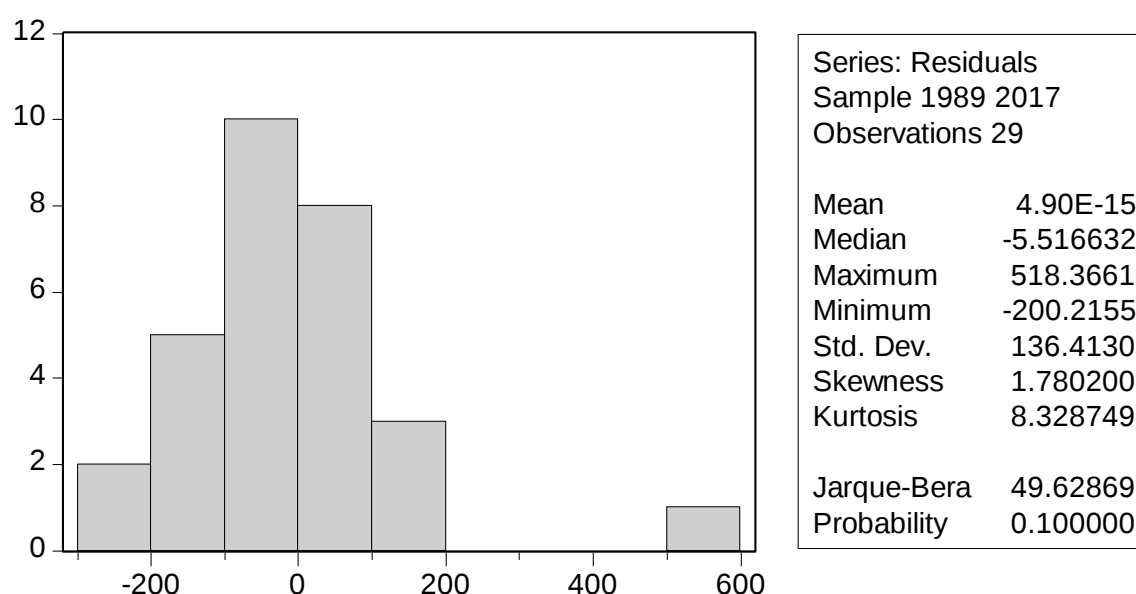
الشكل رقم (05.IV): اختبار التوزيع الطبيعي
