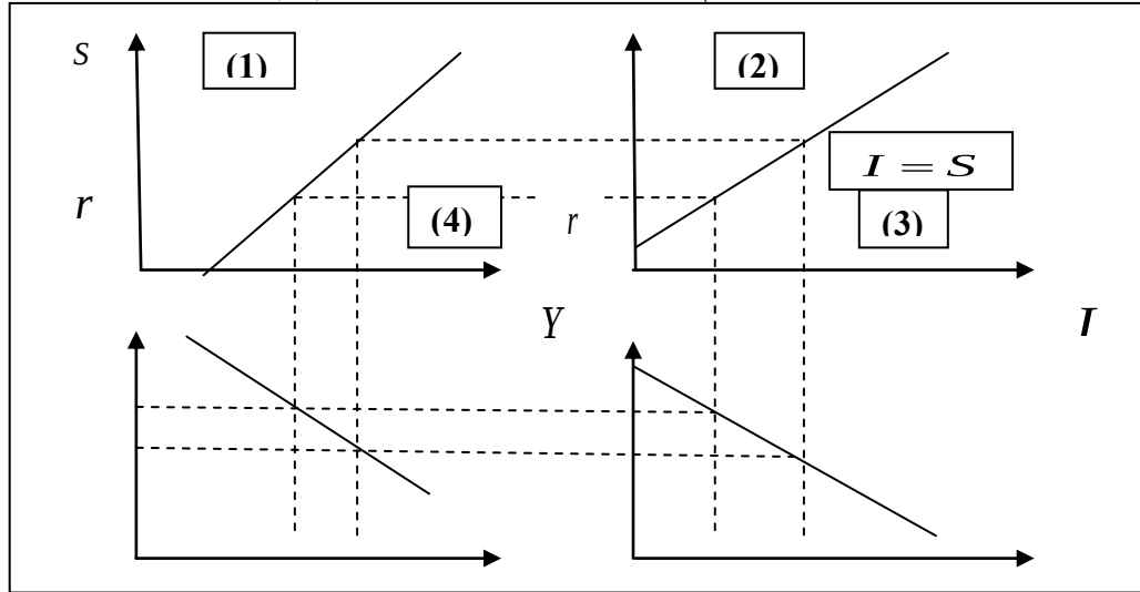
الشكل رقم (II.05): طريقة تحديد المنحنى (IS) بيانيا
