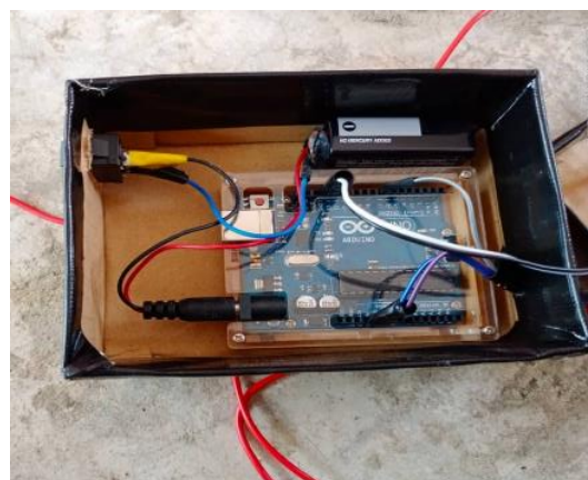
Figure 8 Arduino UNO R3
